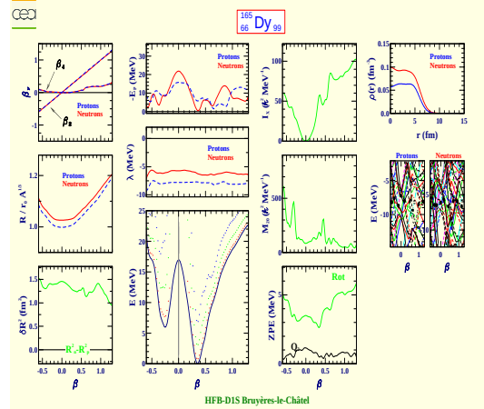
Dysprosium 165 (Z=66, N=99)
