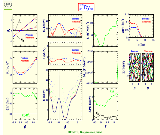
Dysprosium 159 (Z=66, N=93)
