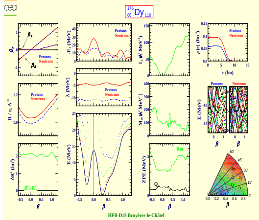
Dysprosium 176 (Z=66, N=110)
