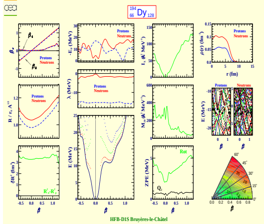
Dysprosium 194 (Z=66, N=128)
