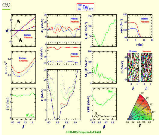
Dysprosium 188 (Z=66, N=122)
