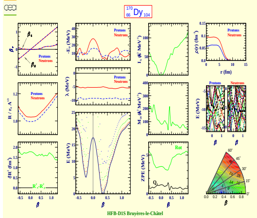
Dysprosium 170 (Z=66, N=104)
