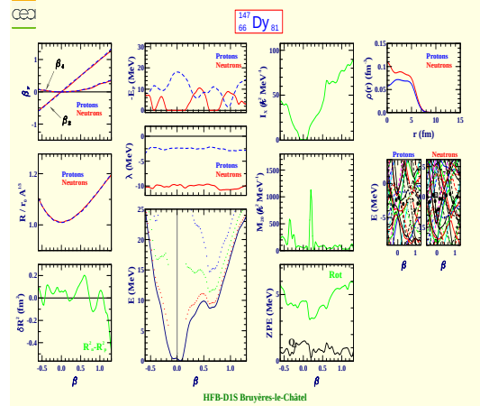
Dysprosium 147 (Z=66, N=81)
