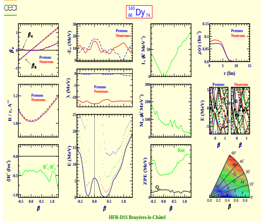
Dysprosium 140 (Z=66, N=74)
