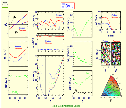
Dysprosium 200 (Z=66, N=134)
