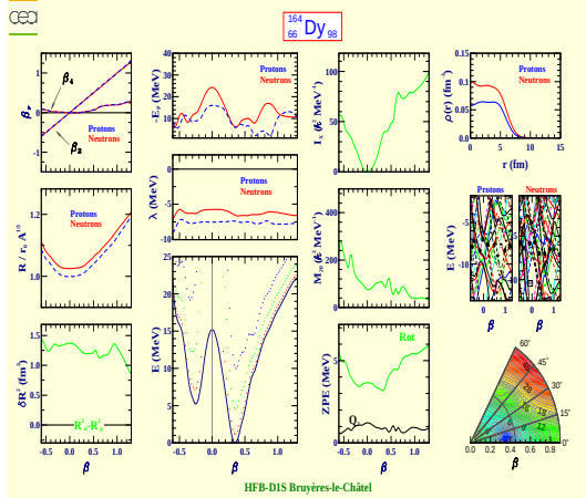
Dysprosium 164 (Z=66, N=98)
