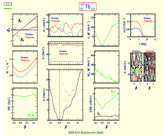
Terbium 197 (Z=65, N=132)
