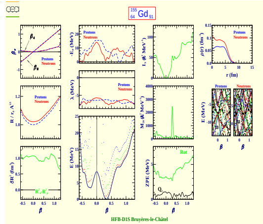
Gadolinium 155 (Z=64, N=91)
