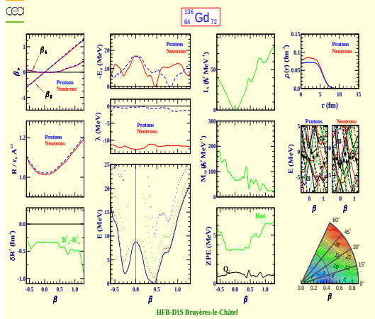
Gadolinium 136 (Z=64, N=72)
