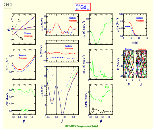
Gadolinium 161 (Z=64, N=97)
