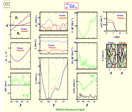
Gadolinium 143 (Z=64, N=79)
