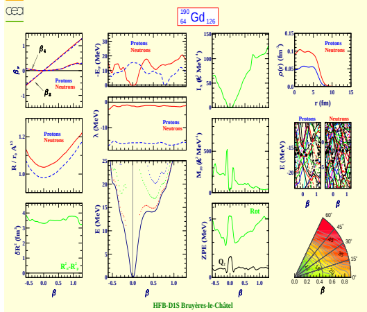
Gadolinium 190 (Z=64, N=126)
