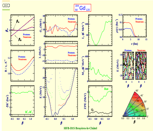
Gadolinium 184 (Z=64, N=120)
