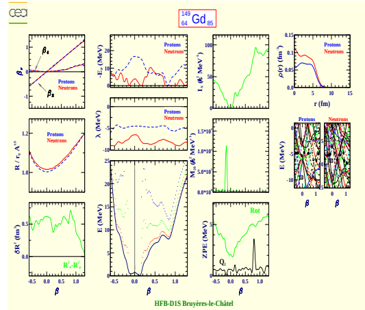
Gadolinium 149 (Z=64, N=85)
