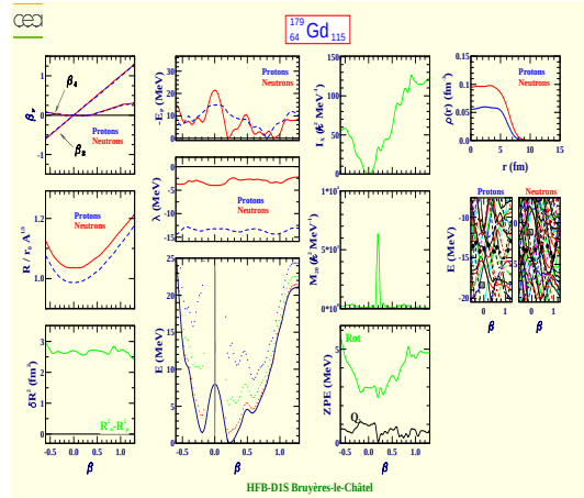
Gadolinium 179 (Z=64, N=115)
