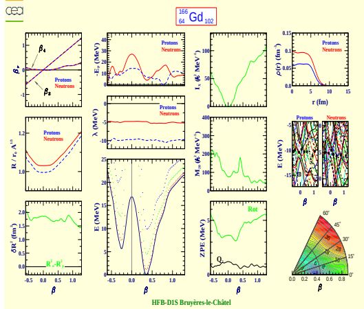
Gadolinium 166 (Z=64, N=102)
