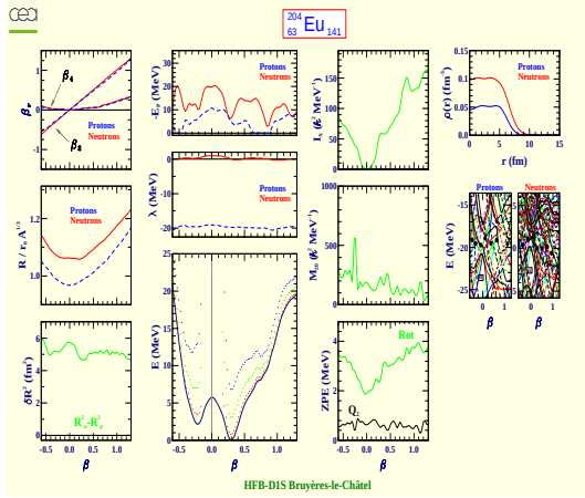
Europium 204 (Z=63, N=141)
