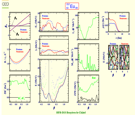
Europium 152 (Z=63, N=89)
