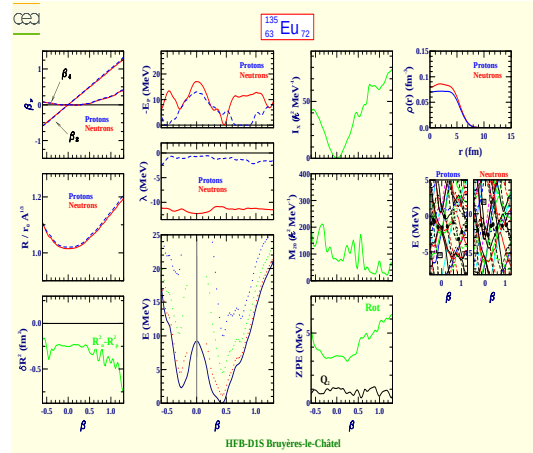
Europium 135 (Z=63, N=72)
