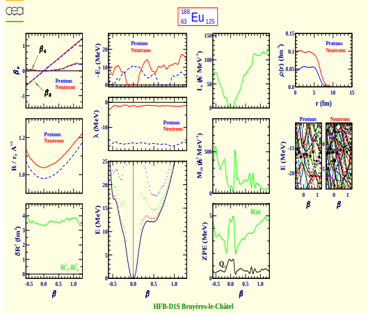
Europium 188 (Z=63, N=125)
