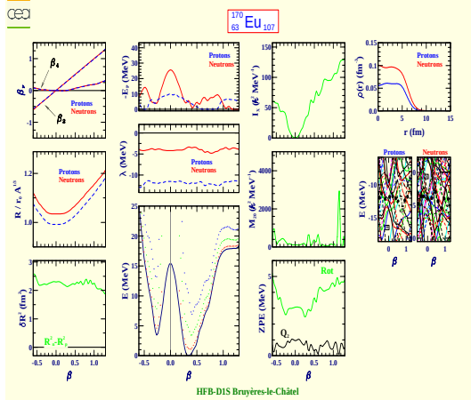
Europium 170 (Z=63, N=107)
