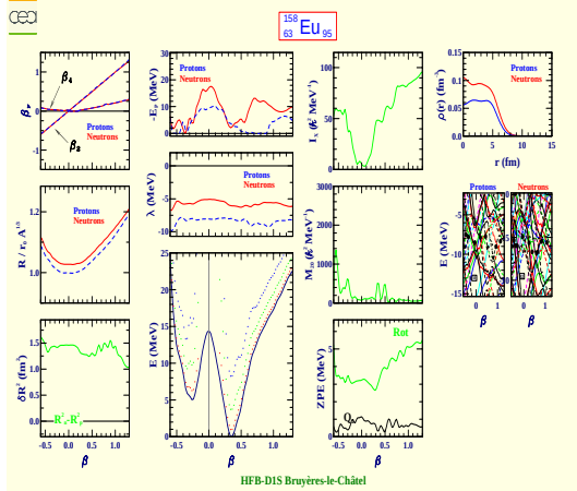
Europium 158 (Z=63, N=95)
