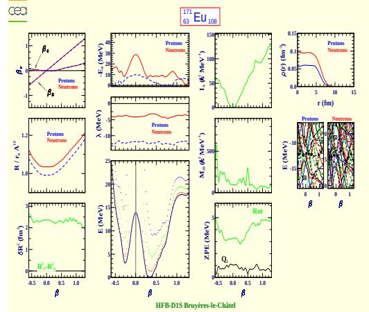
Europium 171 (Z=63, N=108)
