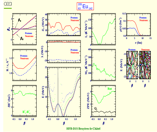
Europium 205 (Z=63, N=142)
