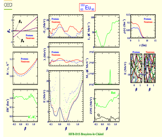
Europium 153 (Z=63, N=90)
