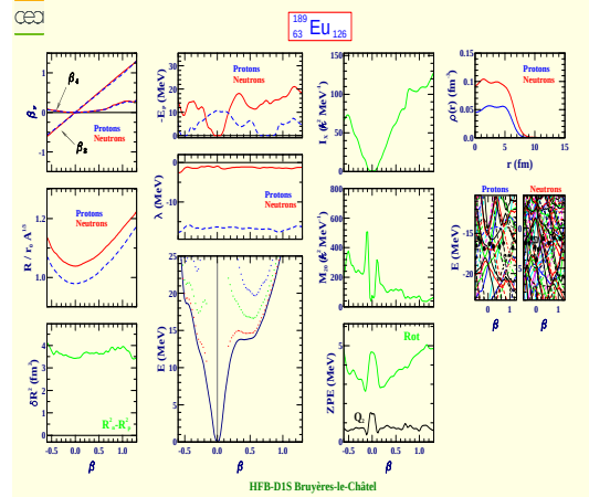
Europium 189 (Z=63, N=126)
