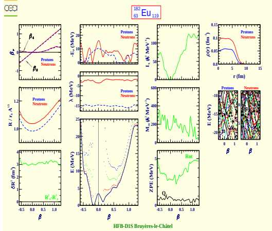
Europium 182 (Z=63, N=119)
