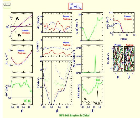
Europium 147 (Z=63, N=84)
