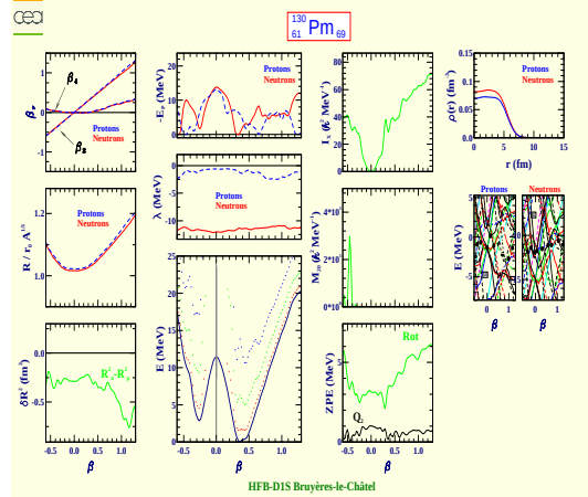
Promethium 130 (Z=61, N=69)
