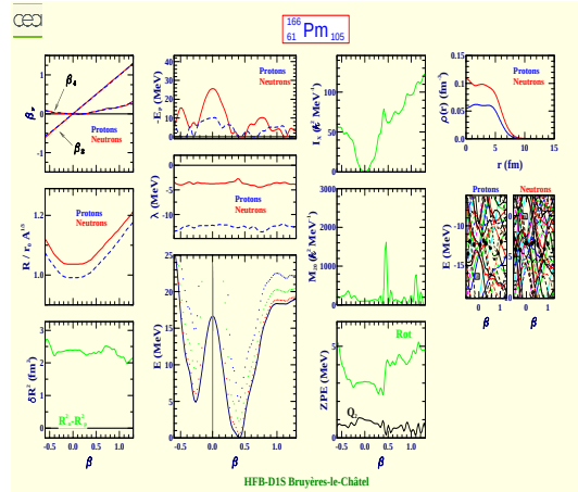
Promethium 166 (Z=61, N=105)
