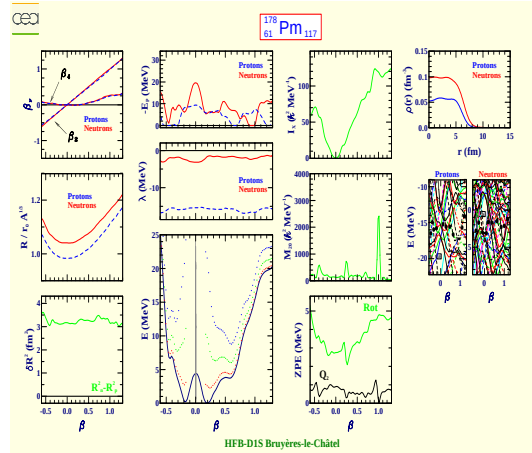
Promethium 178 (Z=61, N=117)
