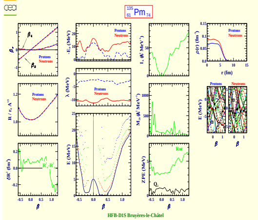
Promethium 135 (Z=61, N=74)
