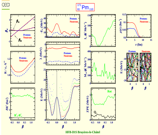
Promethium 171 (Z=61, N=110)
