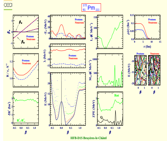
Promethium 172 (Z=61, N=111)
