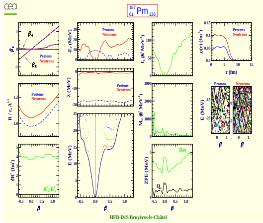
Promethium 187 (Z=61, N=126)
