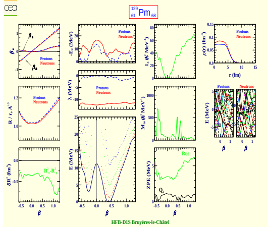
Promethium 129 (Z=61, N=68)
