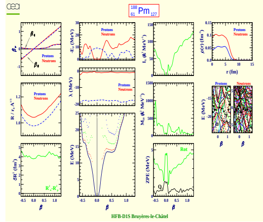
Promethium 188 (Z=61, N=127)
