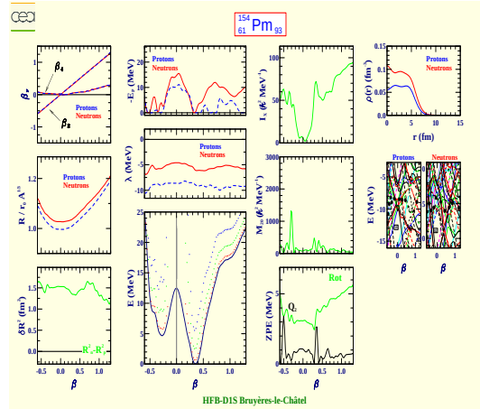
Promethium 154 (Z=61, N=93)
