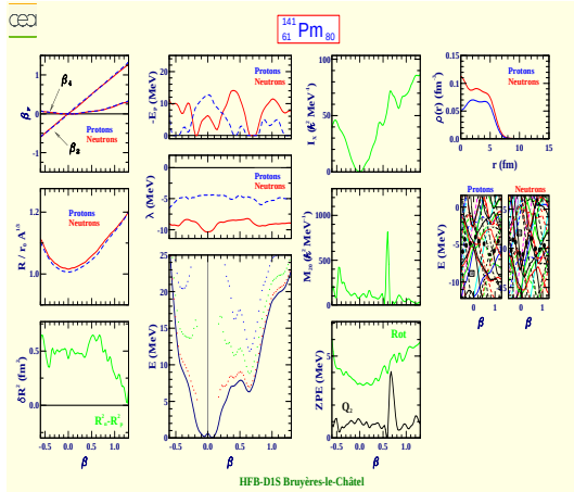
Promethium 141 (Z=61, N=80)
