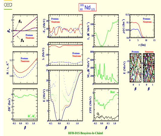
Neodymium 181 (Z=60, N=121)
