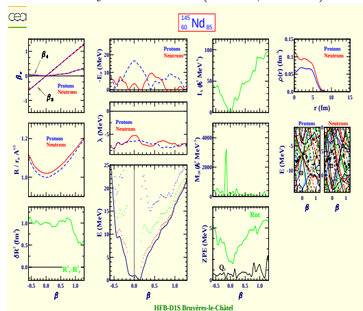
Neodymium 145 (Z=60, N=85)
