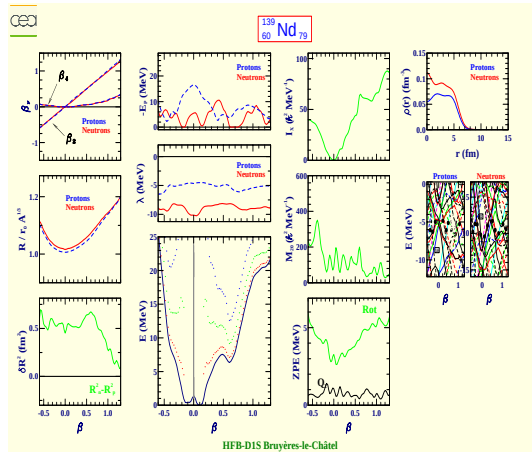
Neodymium 139 (Z=60, N=79)
