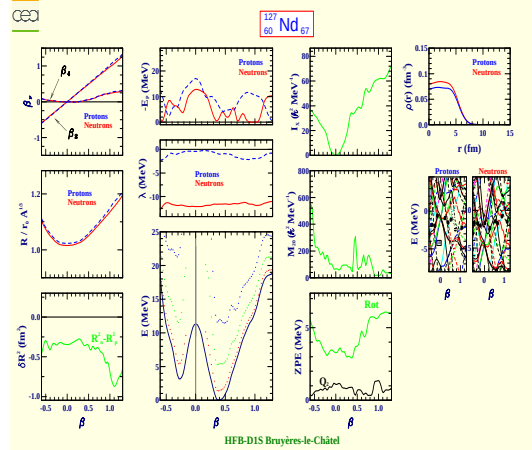
Neodymium 127 (Z=60, N=67)
