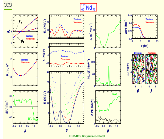
Neodymium 133 (Z=60, N=73)
