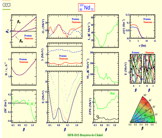
Neodymium 132 (Z=60, N=72)
