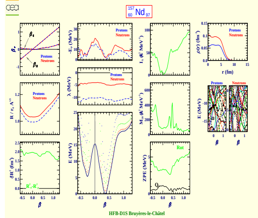
Neodymium 157 (Z=60, N=97)
