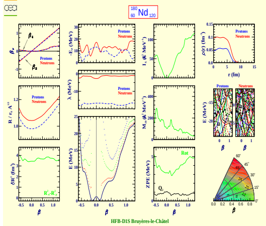
Neodymium 180 (Z=60, N=120)
