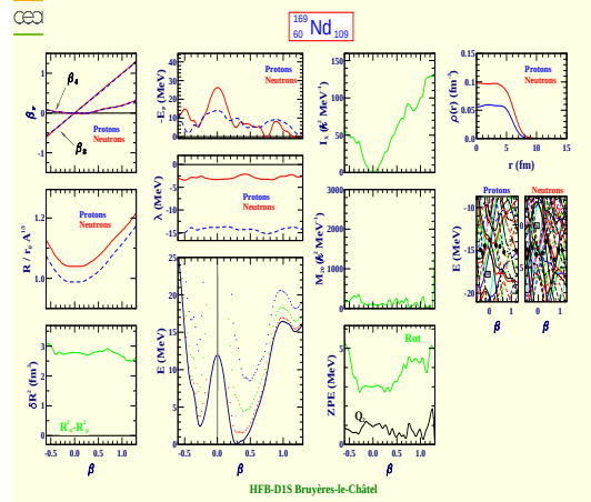
Neodymium 169 (Z=60, N=109)
