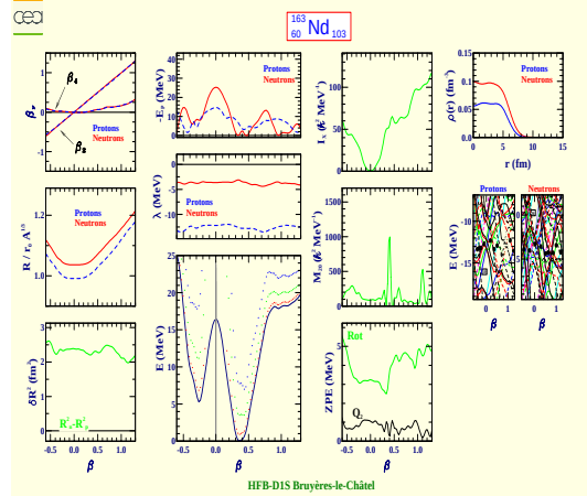
Neodymium 163 (Z=60, N=103)
