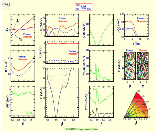
Neodymium 186 (Z=60, N=126)
