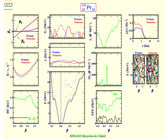
Praseodymium 142 (Z=59, N=83)
