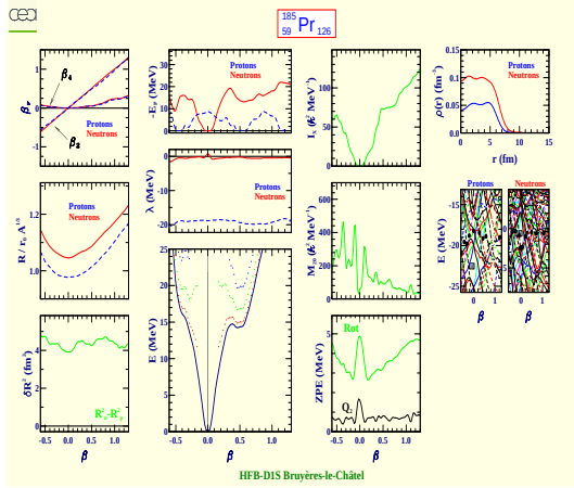
Praseodymium 185 (Z=59, N=126)
