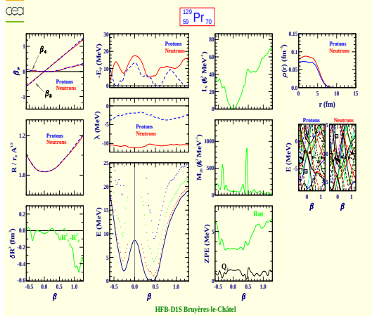
Praseodymium 129 (Z=59, N=70)
