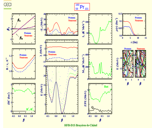
Praseodymium 160 (Z=59, N=101)
