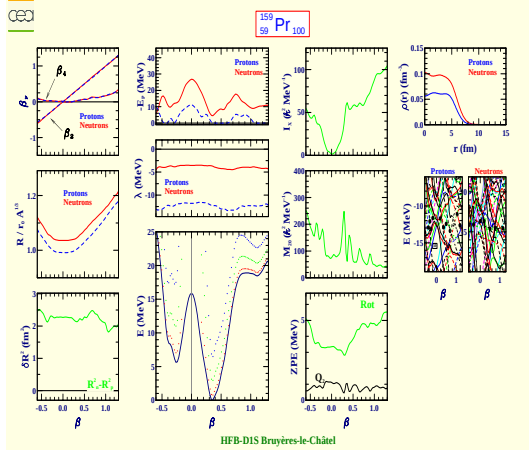
Praseodymium 159 (Z=59, N=100)
