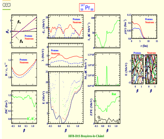
Praseodymium 147 (Z=59, N=88)
