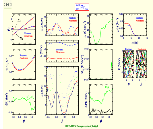
Praseodymium 124 (Z=59, N=65)
