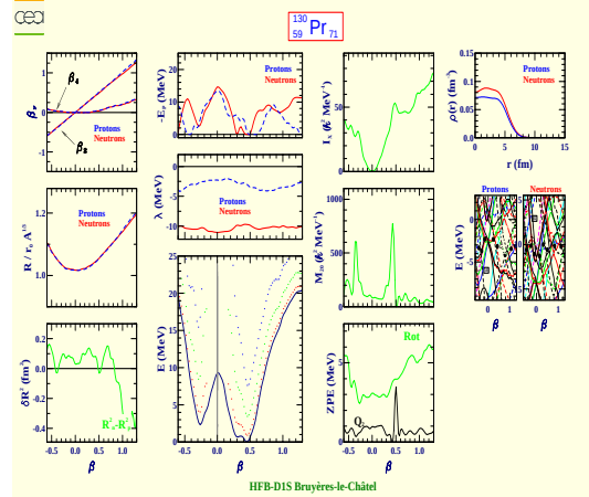
Praseodymium 130 (Z=59, N=71)
