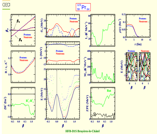
Praseodymium 123 (Z=59, N=64)
