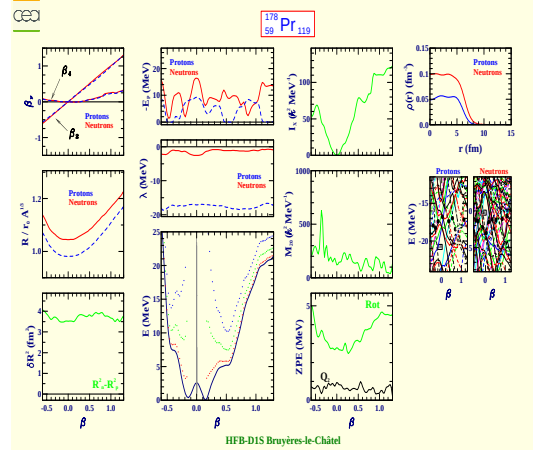
Praseodymium 178 (Z=59, N=119)
