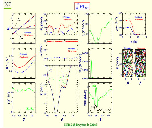
Praseodymium 186 (Z=59, N=127)
