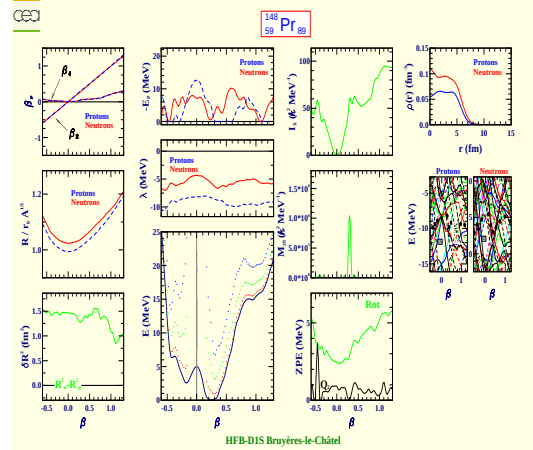
Praseodymium 148 (Z=59, N=89)
