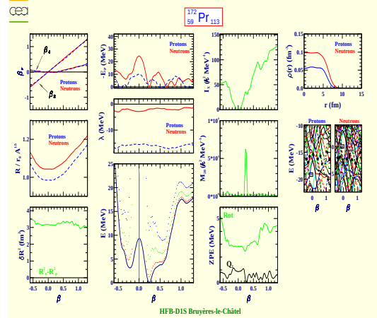
Praseodymium 172 (Z=59, N=113)
