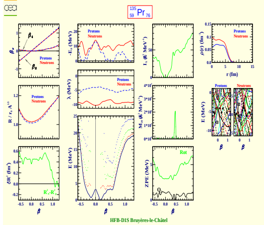
Praseodymium 135 (Z=59, N=76)
