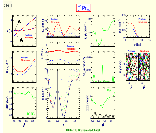
Praseodymium 154 (Z=59, N=95)
