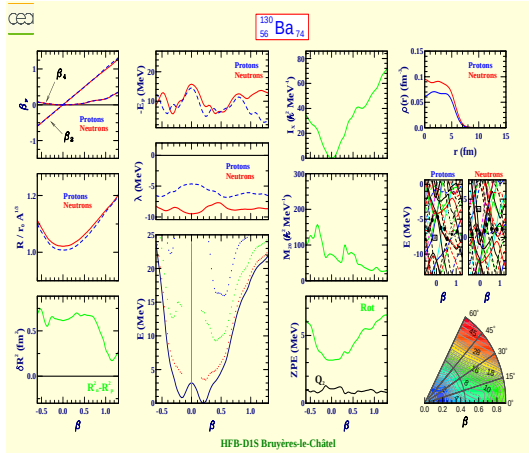
Barium 130 (Z=56, N=74)
