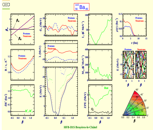
Barium 142 (Z=56, N=86)
