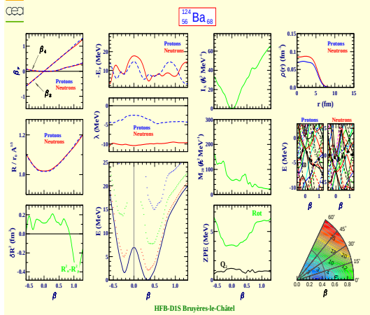
Barium 124 (Z=56, N=68)
