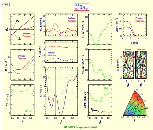
Barium 154 (Z=56, N=98)
