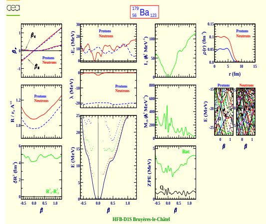
Barium 179 (Z=56, N=123)
