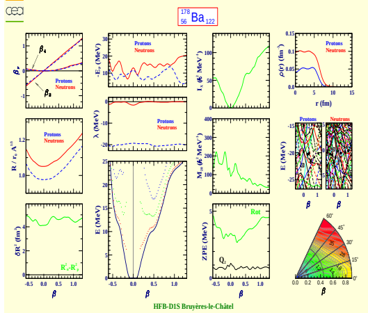
Barium 178 (Z=56, N=122)
