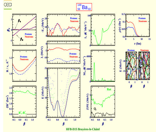
Barium 149 (Z=56, N=93)
