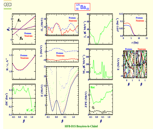
Barium 125 (Z=56, N=69)
