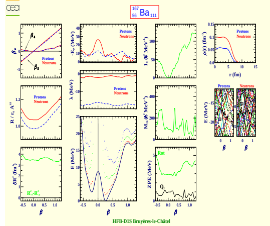
Barium 167 (Z=56, N=111)
