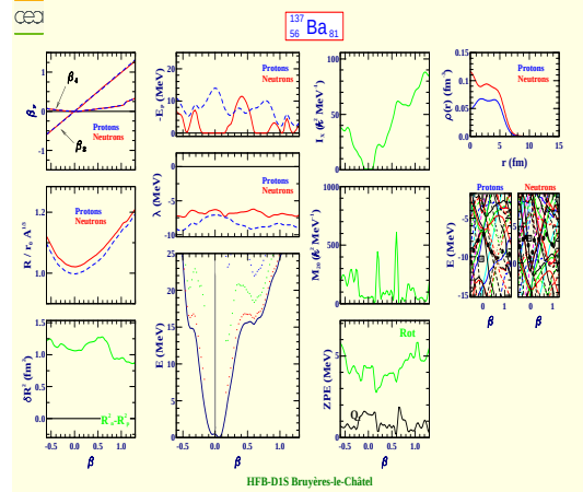
Barium 137 (Z=56, N=81)
