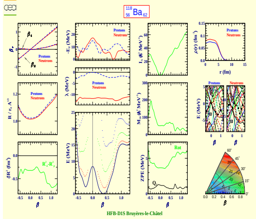
Barium 118 (Z=56, N=62)
