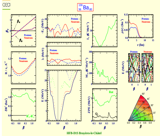
Barium 136 (Z=56, N=80)
