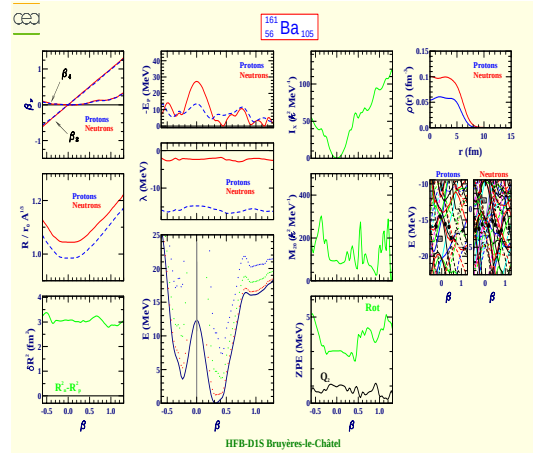
Barium 161 (Z=56, N=105)
