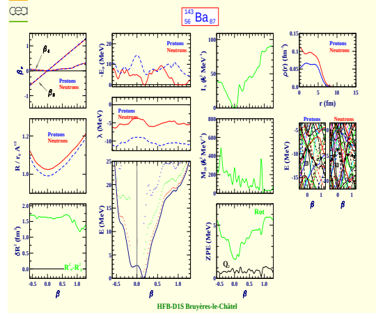
Barium 143 (Z=56, N=87)
