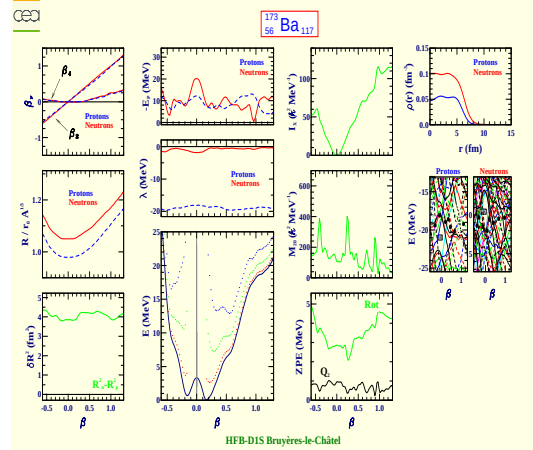
Barium 173 (Z=56, N=117)
