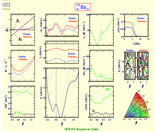
Barium 148 (Z=56, N=92)
