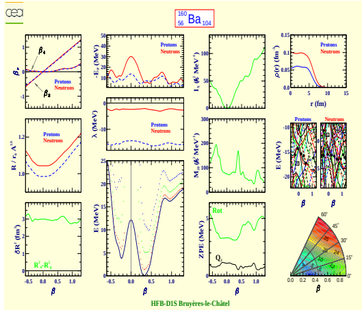
Barium 160 (Z=56, N=104)
