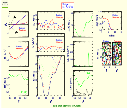
Cesium 134 (Z=55, N=79)
