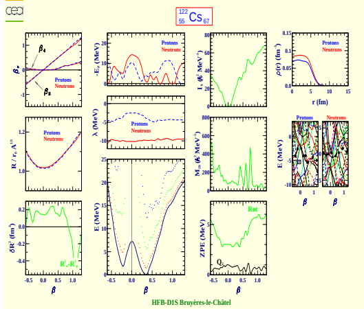
Cesium 122 (Z=55, N=67)
