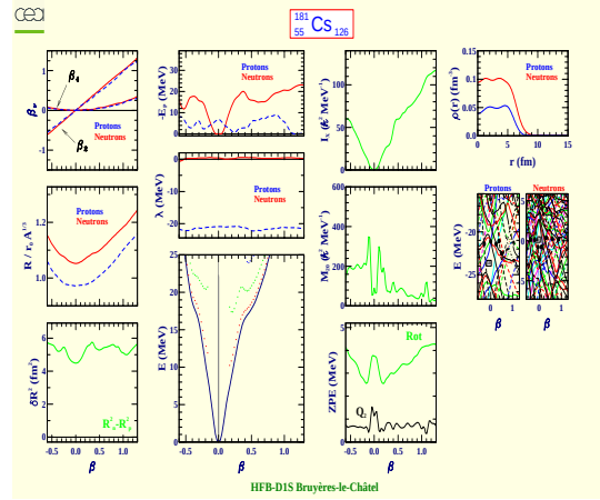
Cesium 181 (Z=55, N=126)
