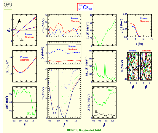
Cesium 123 (Z=55, N=68)
