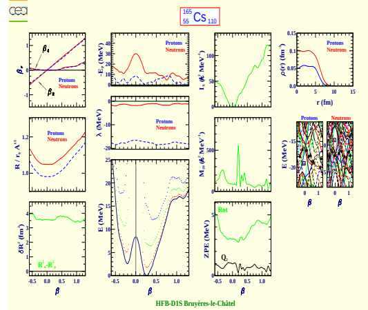
Cesium 165 (Z=55, N=110)
