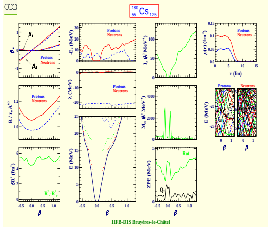
Cesium 180 (Z=55, N=125)
