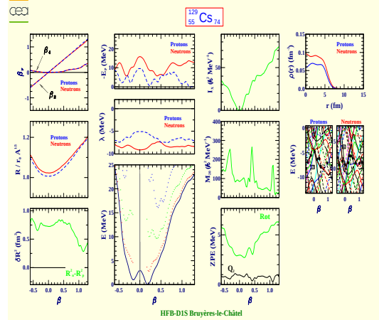
Cesium 129 (Z=55, N=74)
