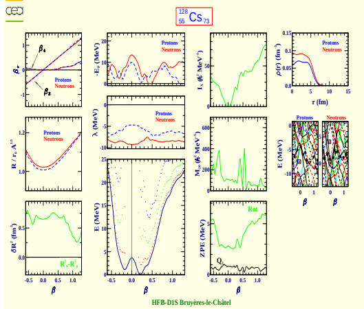
Cesium 128 (Z=55, N=73)
