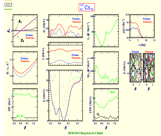
Cesium 147 (Z=55, N=92)
