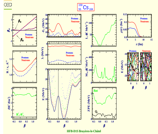
Cesium 159 (Z=55, N=104)
