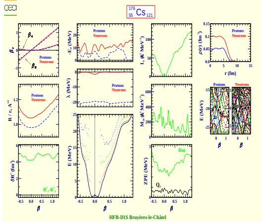
Cesium 176 (Z=55, N=121)
