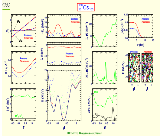
Cesium 158 (Z=55, N=103)
