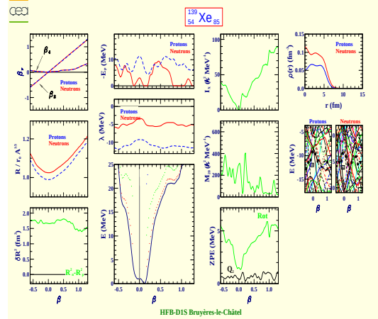
Xenon 139 (Z=54, N=85)
