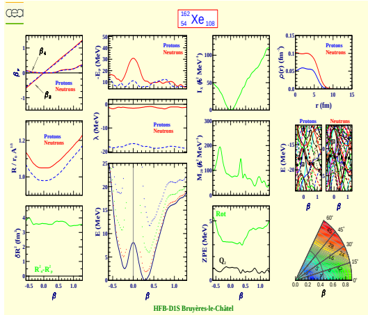
Xenon 162 (Z=54, N=108)
