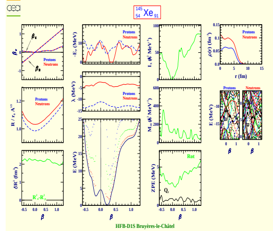
Xenon 145 (Z=54, N=91)
