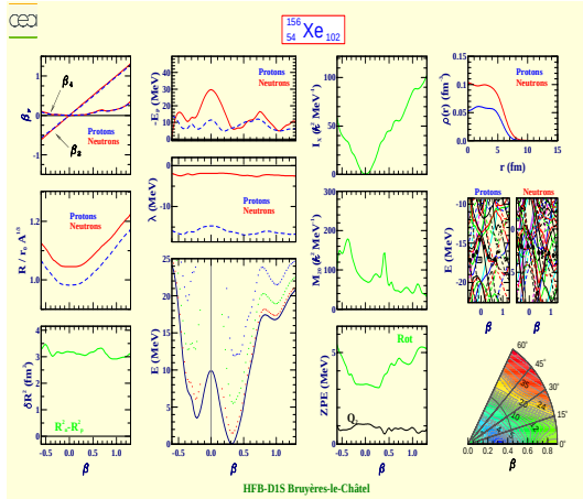
Xenon 156 (Z=54, N=102)
