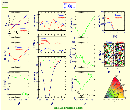
Xenon 138 (Z=54, N=84)
