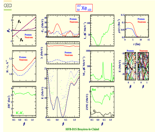
Xenon 157 (Z=54, N=103)
