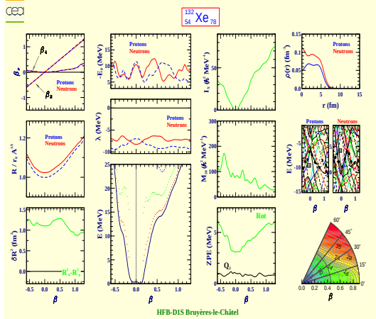
Xenon 132 (Z=54, N=78)
