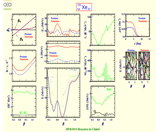
Xenon 151 (Z=54, N=97)
