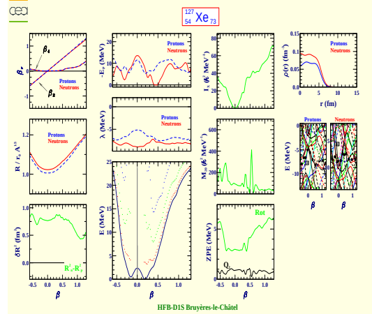
Xenon 127 (Z=54, N=73)
