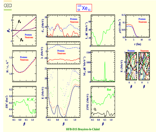
Xenon 115 (Z=54, N=61)
