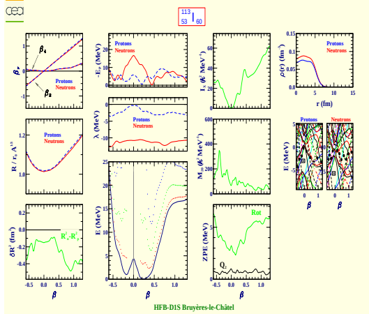
Iodine 113 (Z=53, N=60)
