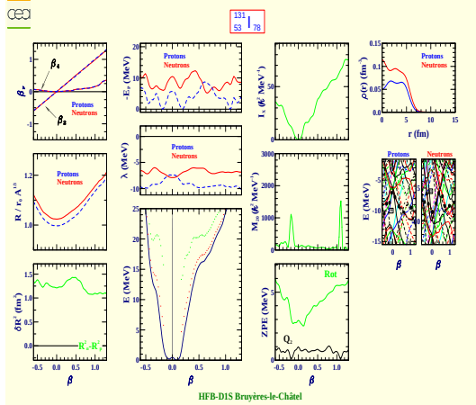
Iodine 131 (Z=53, N=78)
