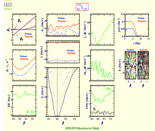
Iodine 174 (Z=53, N=121)
