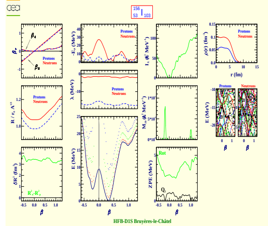
Iodine 156 (Z=53, N=103)
