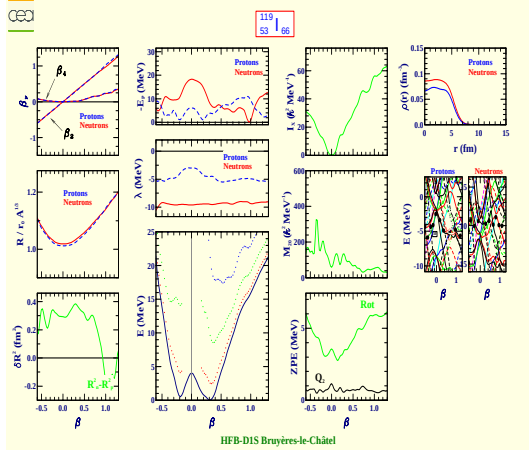
Iodine 119 (Z=53, N=66)
