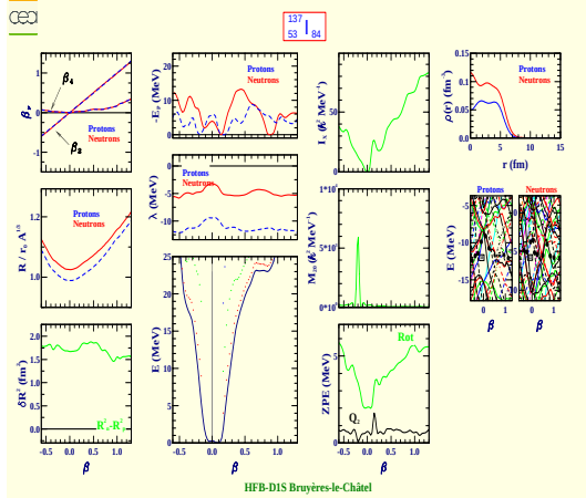
Iodine 137 (Z=53, N=84)
