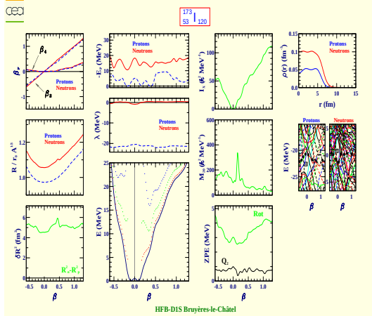
Iodine 173 (Z=53, N=120)
