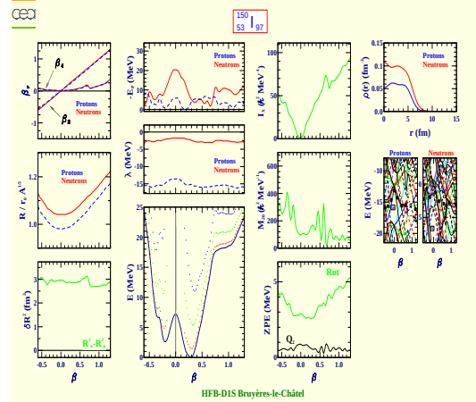
Iodine 150 (Z=53, N=97)
