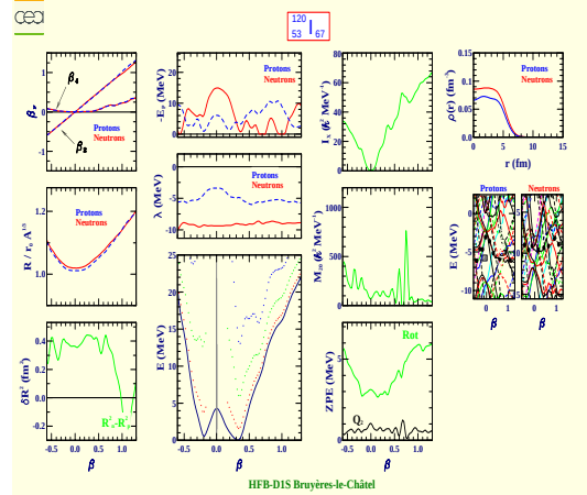
Iodine 120 (Z=53, N=67)
