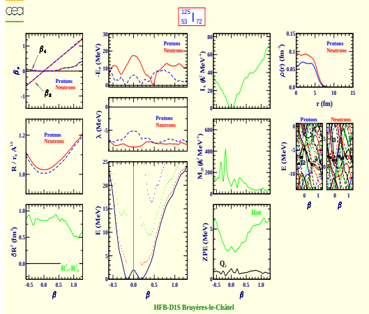
Iodine 125 (Z=53, N=72)
