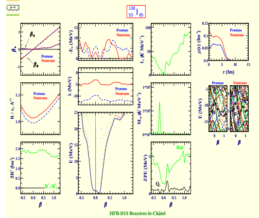
Iodine 138 (Z=53, N=85)
