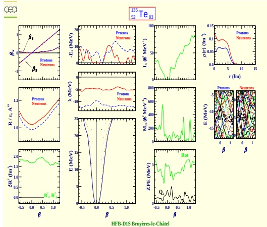
Tellure 135 (Z=52, N=83)
