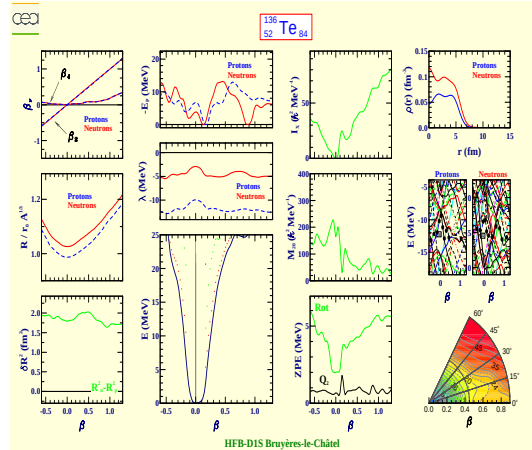
Tellure 136 (Z=52, N=84)
