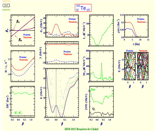
Tellure 159 (Z=52, N=107)
