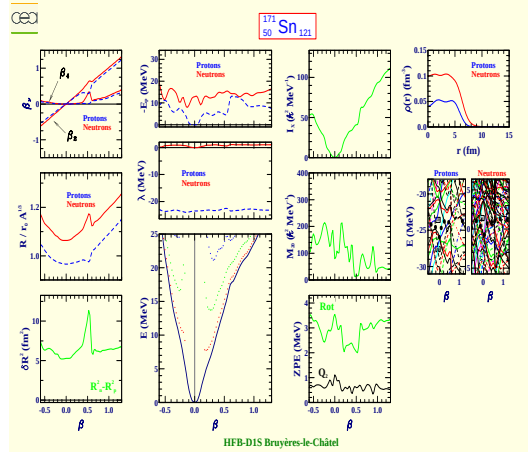
Tin 171 (Z=50, N=121)
