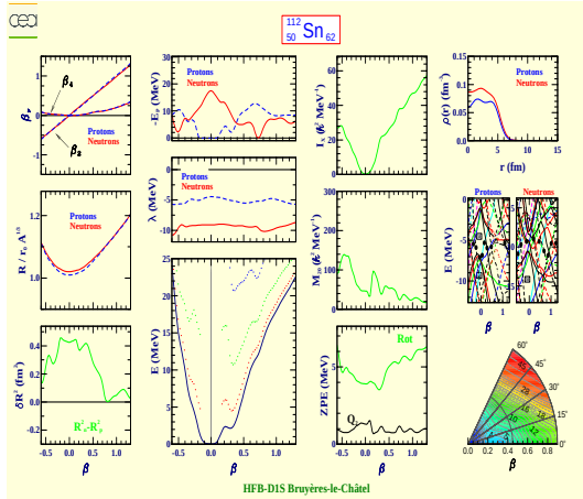
Tin 112 (Z=50, N=62)
