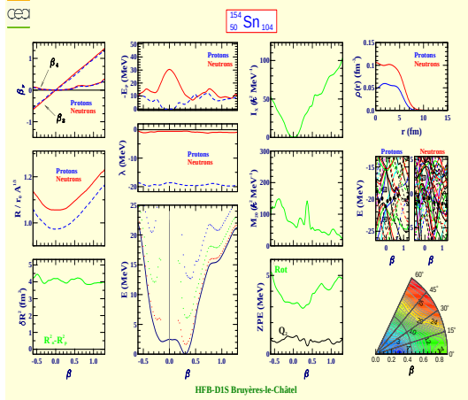
Tin 154 (Z=50, N=104)
