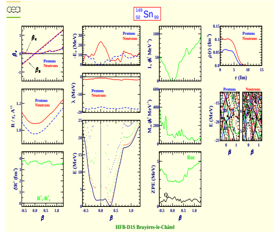
Tin 149 (Z=50, N=99)
