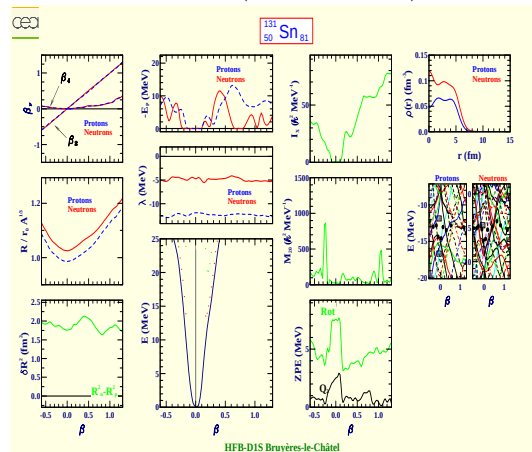
Tin 131 (Z=50, N=81)
