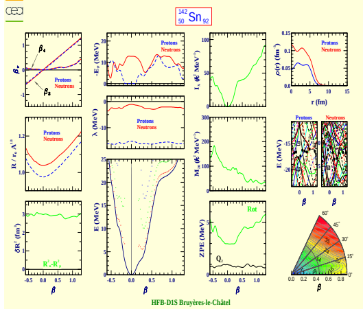
Tin 142 (Z=50, N=92)
