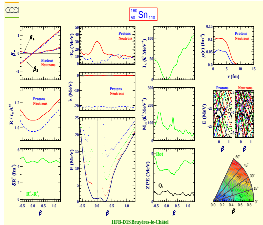
Tin 160 (Z=50, N=110)
