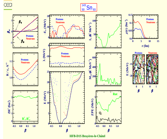
Tin 143 (Z=50, N=93)
