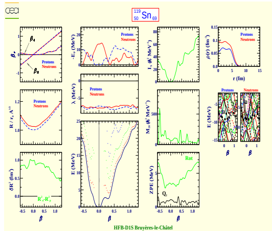
Tin 119 (Z=50, N=69)
