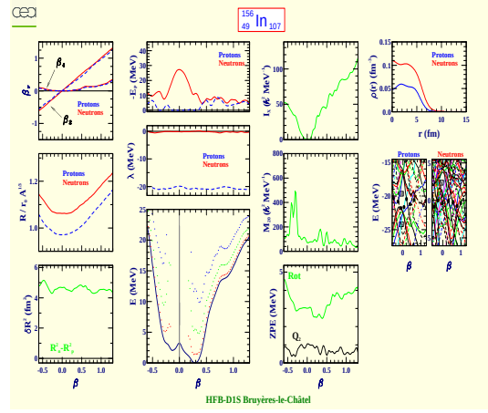
Indium 156 (Z=49, N=107)
