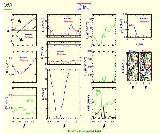
Indium 100 (Z=49, N=51)
