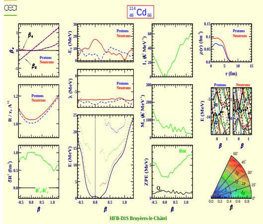
Cadmium 114 (Z=48, N=66)
