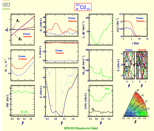
Cadmium 150 (Z=48, N=102)
