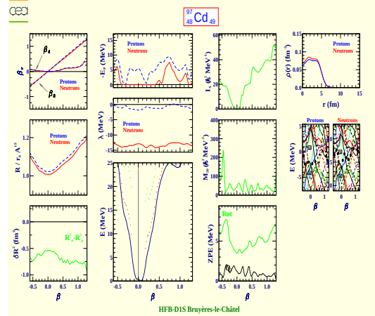
Cadmium 97 (Z=48, N=49)
