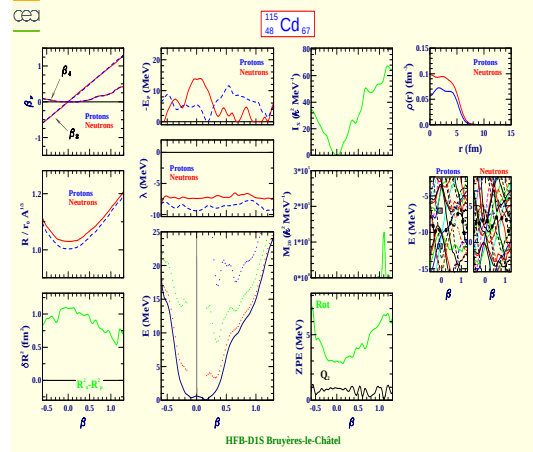
Cadmium 115 (Z=48, N=67)
