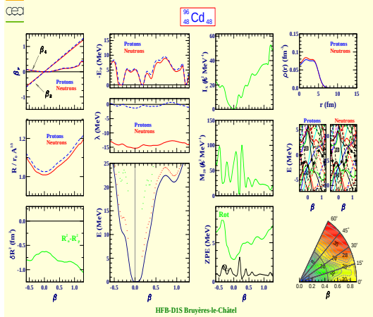
Cadmium 96 (Z=48, N=48)
