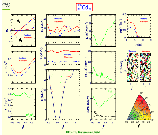
Cadmium 126 (Z=48, N=78)
