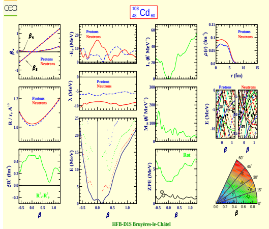
Cadmium 108 (Z=48, N=60)
