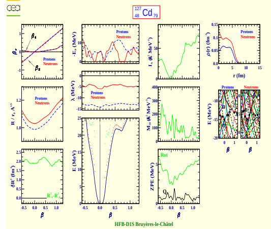
Cadmium 127 (Z=48, N=79)
