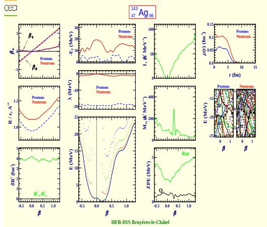
Silver 143 (Z=47, N=96)
