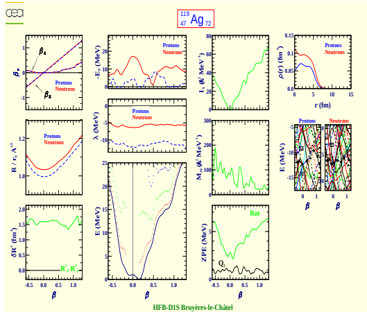
Silver 119 (Z=47, N=72)
