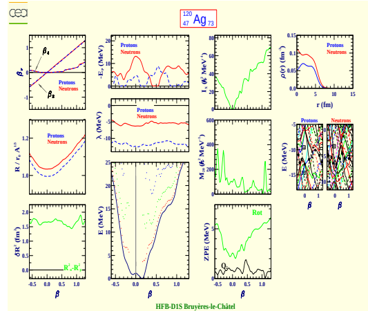
Silver 120 (Z=47, N=73)
