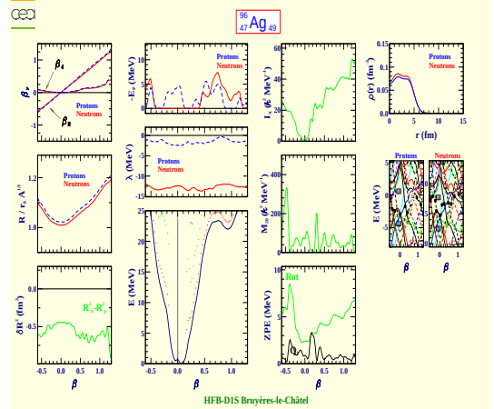
Silver 96 (Z=47, N=49)
