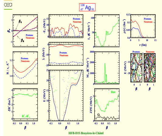
Silver 138 (Z=47, N=91)
