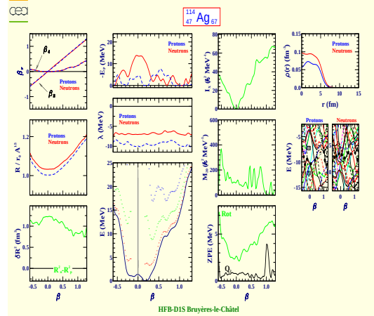
Silver 114 (Z=47, N=67)
