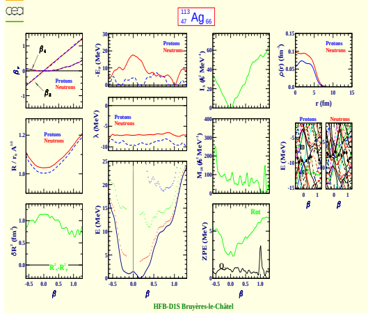
Argent 113 (Z=47, N=66)
