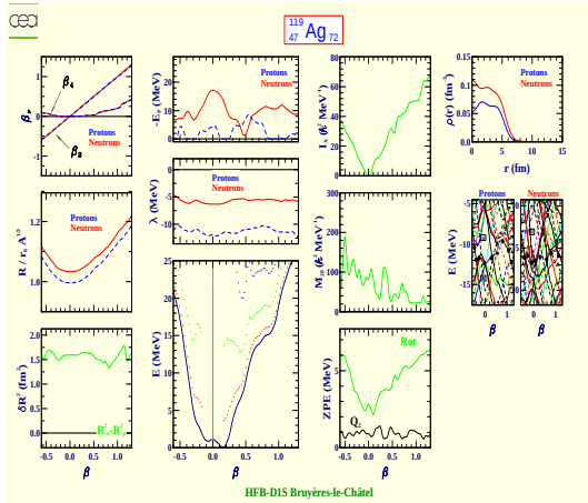
Argent 119 (Z=47, N=72)
