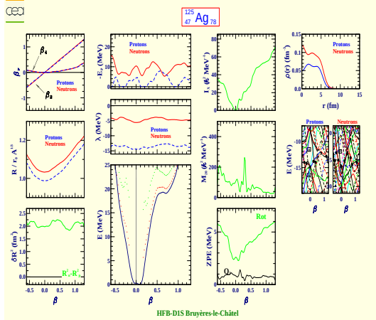
Argent 125 (Z=47, N=78)
