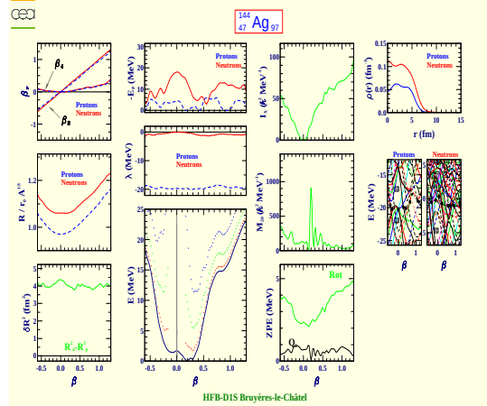
Argent 144 (Z=47, N=97)
