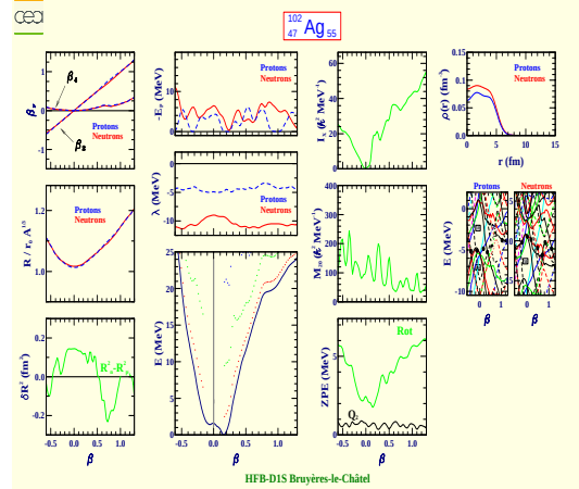
Argent 102 (Z=47, N=55)
