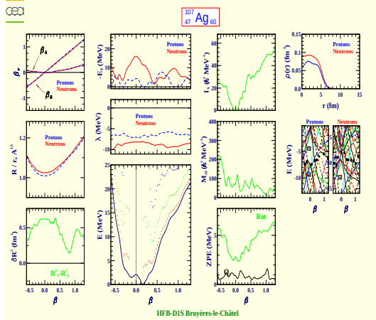
Argent 107 (Z=47, N=60)
