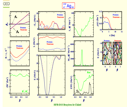
Argent 132 (Z=47, N=85)
