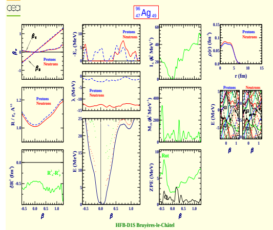
Argent 96 (Z=47, N=49)
