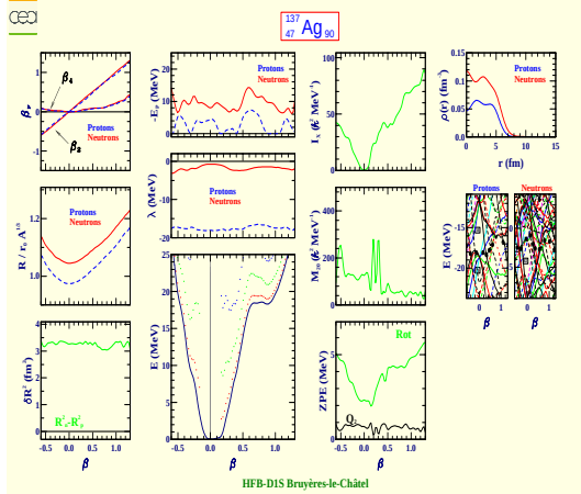
Argent 137 (Z=47, N=90)
