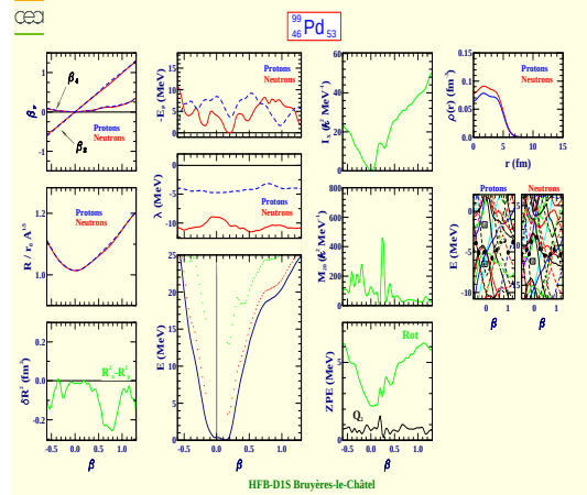
Palladium 99 (Z=46, N=53)
