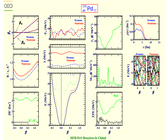
Palladium 123 (Z=46, N=77)
