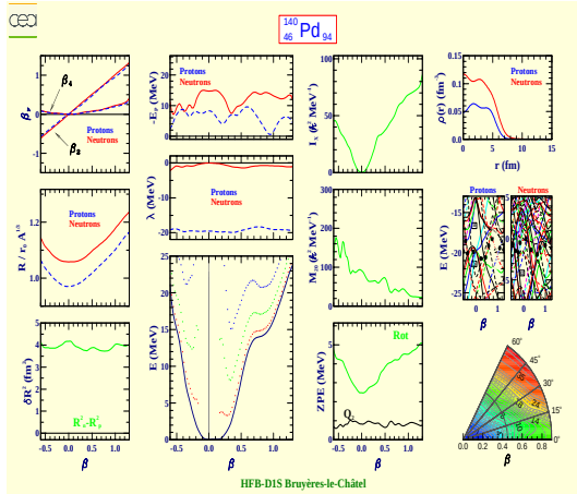
Palladium 140 (Z=46, N=94)
