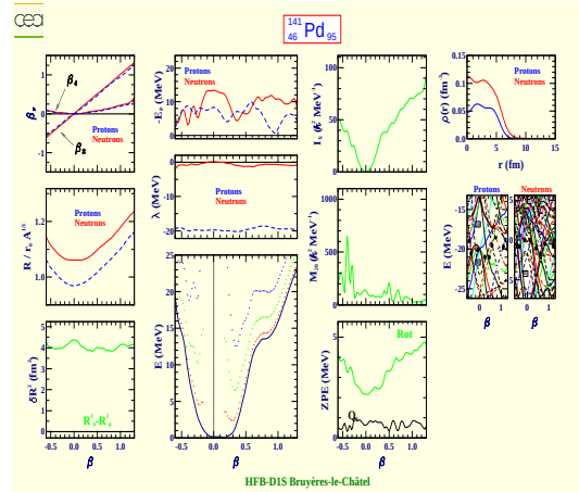
Palladium 141 (Z=46, N=95)
