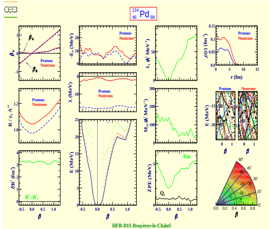
Palladium 134 (Z=46, N=88)
