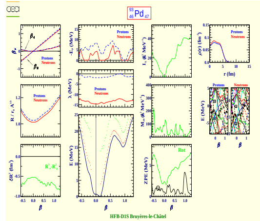
Palladium 93 (Z=46, N=47)
