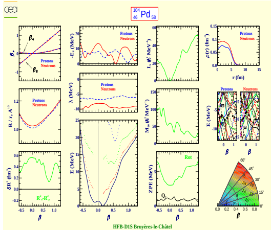
Palladium 104 (Z=46, N=58)
