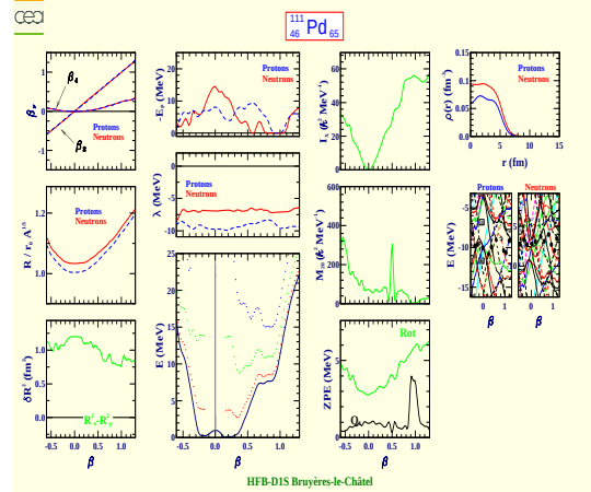
Palladium 111 (Z=46, N=65)
