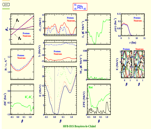
Rhodium 91 (Z=45, N=46)
