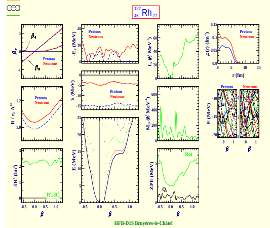
Rhodium 122 (Z=45, N=77)
