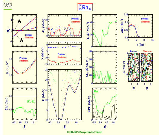
Rhodium 92 (Z=45, N=47)
