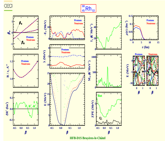
Rhodium 98 (Z=45, N=53)
