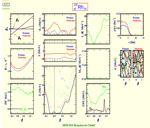
Rhodium 109 (Z=45, N=64)
