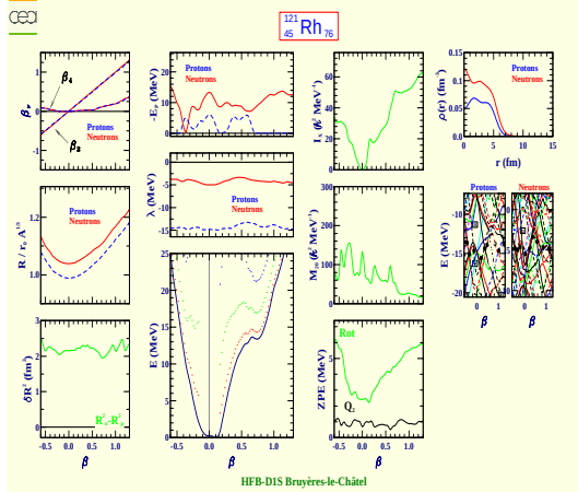
Rhodium 121 (Z=45, N=76)
