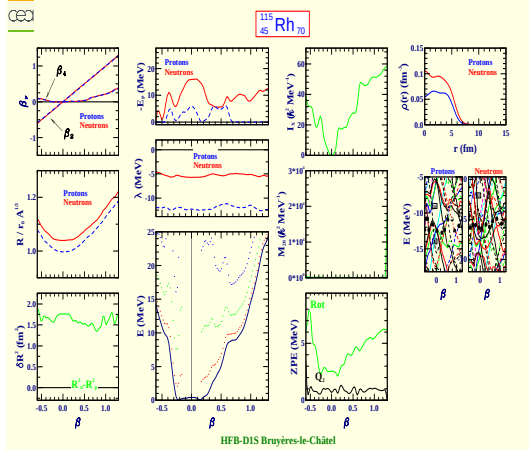
Rhodium 115 (Z=45, N=70)
