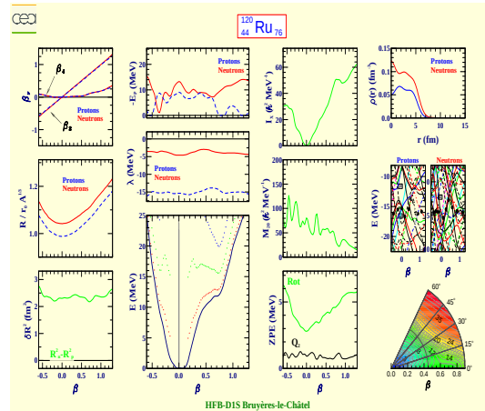
Ruthénium 120 (Z=44, N=76)
