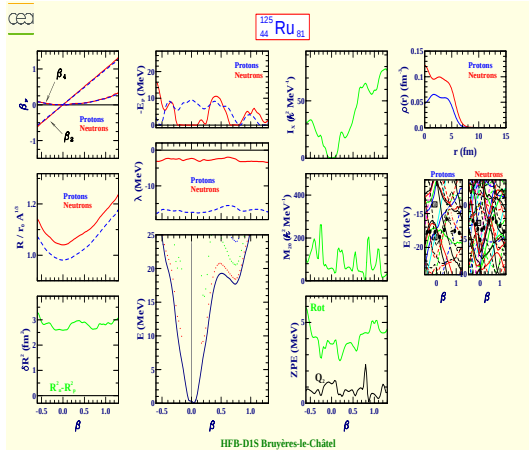
Ruthénium 125 (Z=44, N=81)
