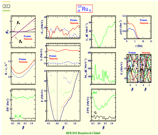
Ruthénium 119 (Z=44, N=75)
