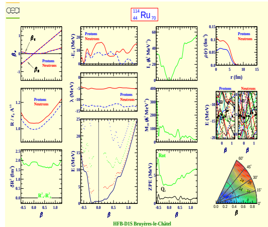
Ruthénium 114 (Z=44, N=70)
