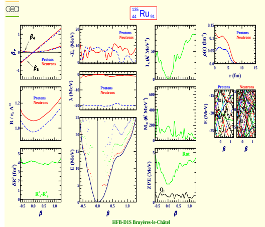
Ruthénium 135 (Z=44, N=91)
