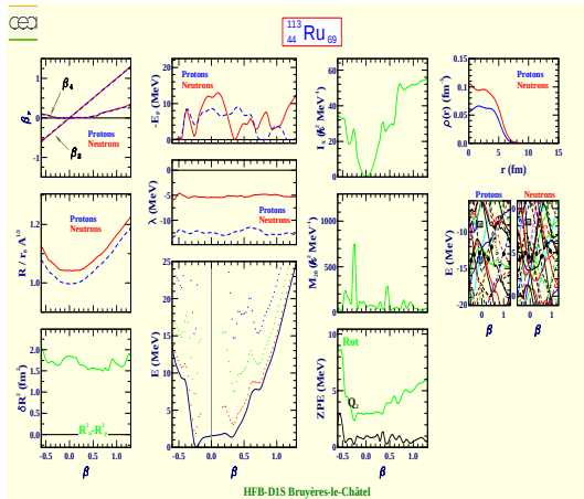
Ruthénium 113 (Z=44, N=69)
