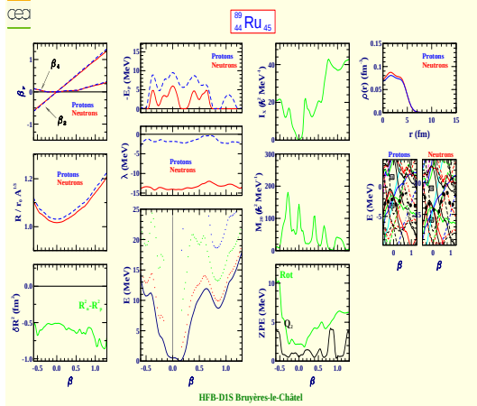
Ruthénium 89 (Z=44, N=45)
