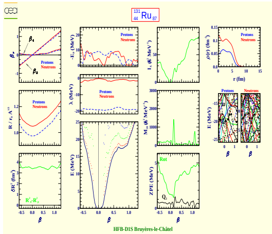
Ruthénium 131 (Z=44, N=87)
