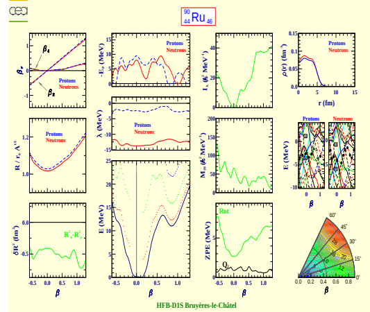
Ruthénium 90 (Z=44, N=46)
