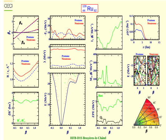
Ruthénium 126 (Z=44, N=82)
