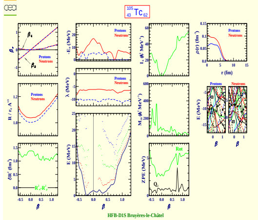
Technetium 105 (Z=43, N=62)
