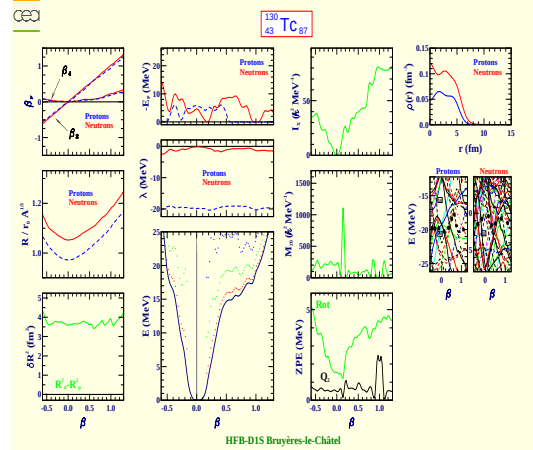
Technetium 130 (Z=43, N=87)
