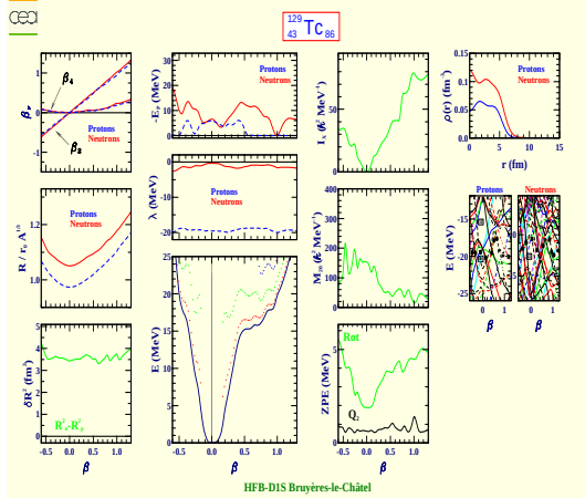
Technetium 129 (Z=43, N=86)
