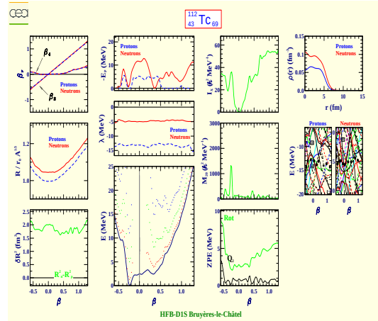
Technetium 112 (Z=43, N=69)
