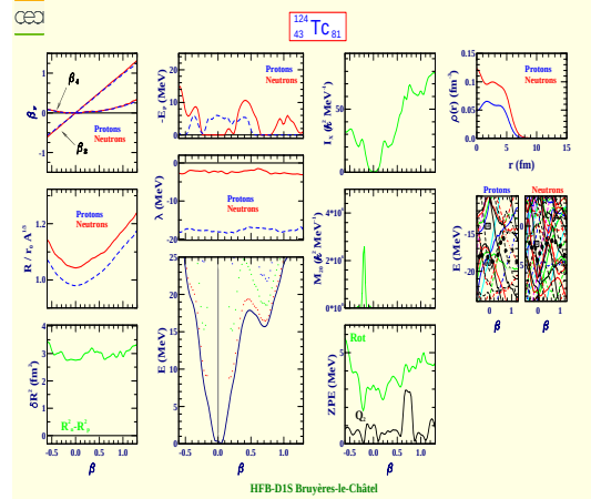
Technetium 124 (Z=43, N=81)
