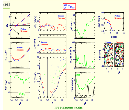
Technetium 100 (Z=43, N=57)
