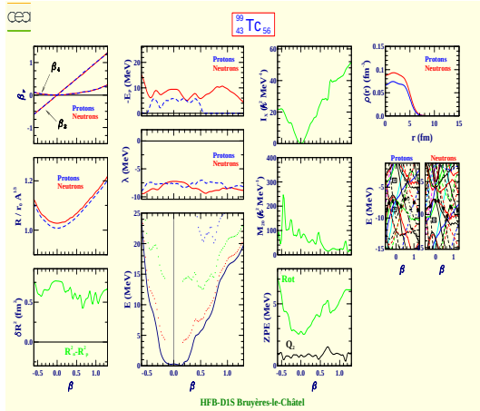
Technetium 99 (Z=43, N=56)
