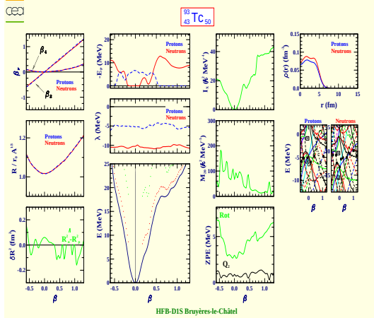
Technetium 93 (Z=43, N=50)
