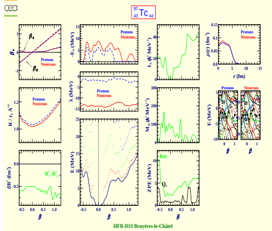
Technetium 87 (Z=43, N=44)
