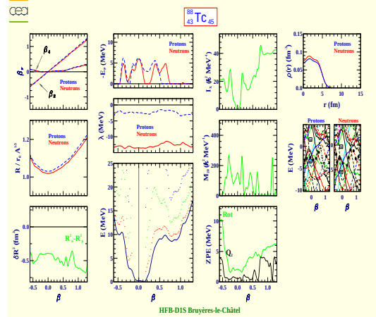
Technetium 88 (Z=43, N=45)
