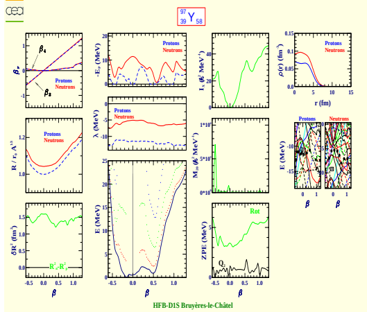
Yttrium 97 (Z=39, N=58)
