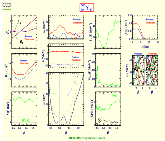
Yttrium 103 (Z=39, N=64)
