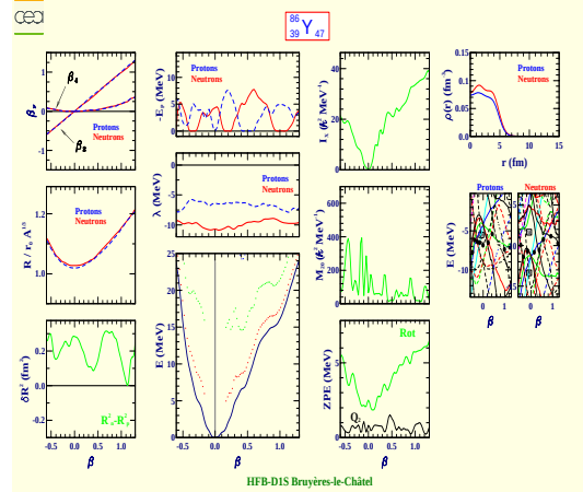
Yttrium 86 (Z=39, N=47)
