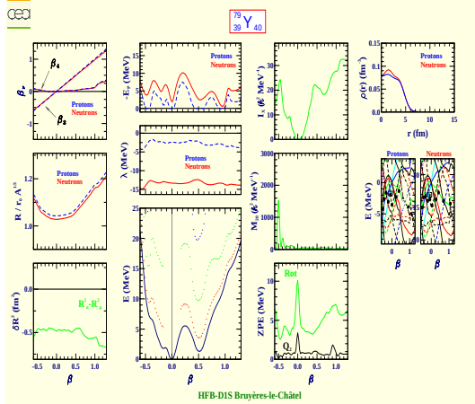
Yttrium 79 (Z=39, N=40)
