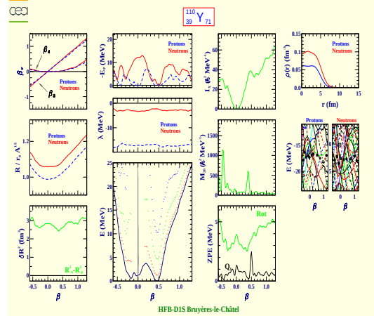
Yttrium 110 (Z=39, N=71)
