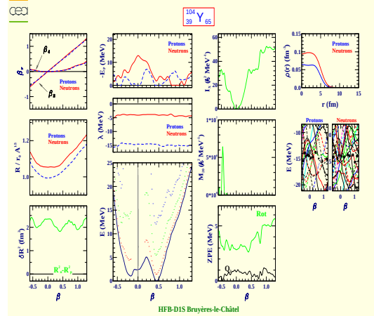
Yttrium 104 (Z=39, N=65)
