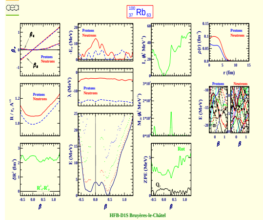
Rubidium 100 (Z=37, N=63)
