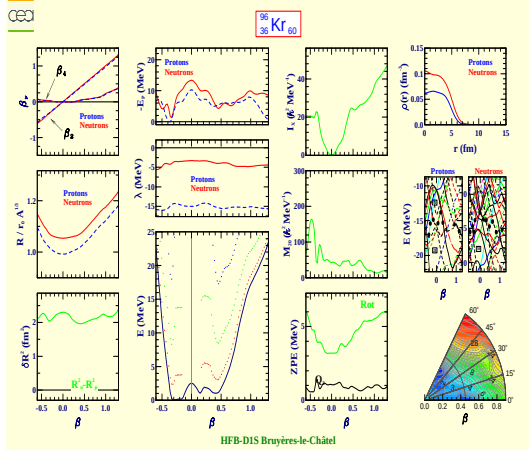
Krypton 96 (Z=36, N=60)
