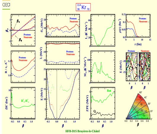
Krypton 114 (Z=36, N=78)
