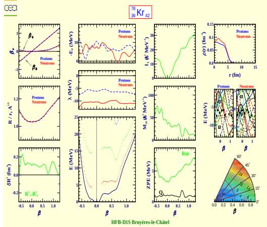
Krypton 78 (Z=36, N=42)
