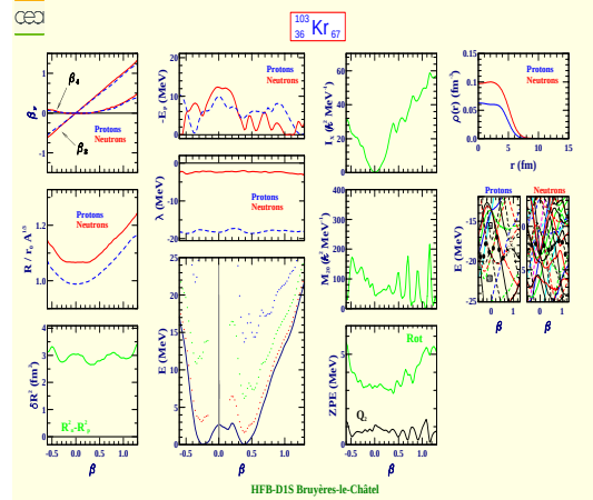
Krypton 103 (Z=36, N=67)
