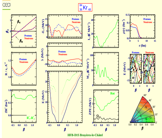
Krypton 84 (Z=36, N=48)
