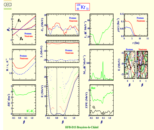
Krypton 109 (Z=36, N=73)
