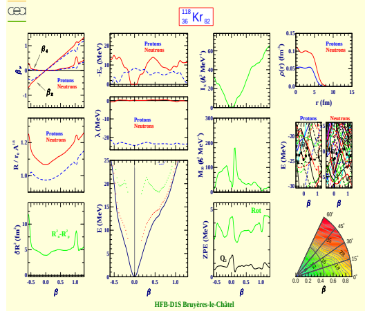
Krypton 118 (Z=36, N=82)
