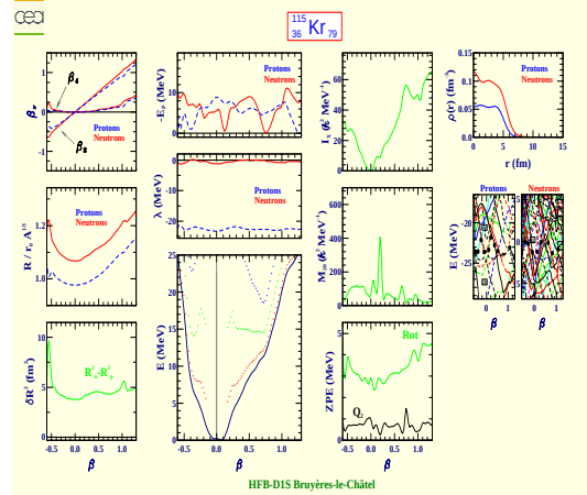
Krypton 115 (Z=36, N=79)
