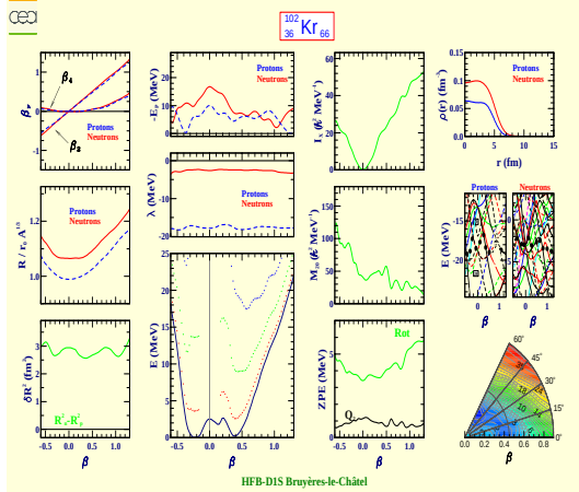
Krypton 102 (Z=36, N=66)
