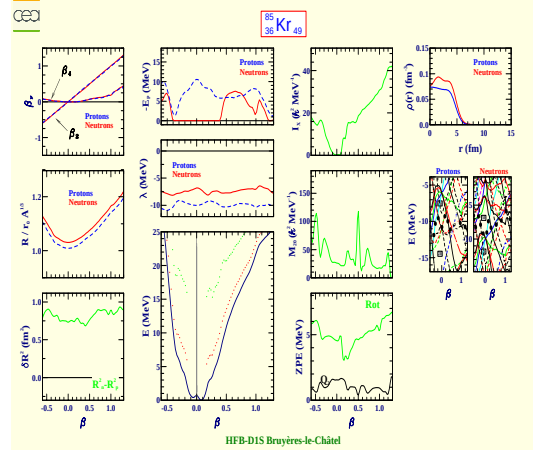
Krypton 85 (Z=36, N=49)
