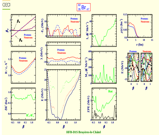
Bromine 82 (Z=35, N=47)
