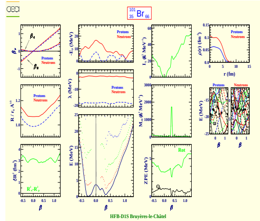
Bromine 101 (Z=35, N=66)
