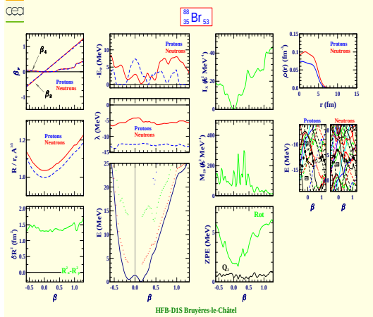
Bromine 88 (Z=35, N=53)
