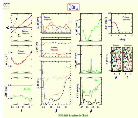
Bromine 71 (Z=35, N=36)
