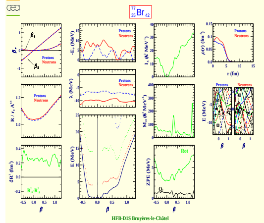
Bromine 77 (Z=35, N=42)
