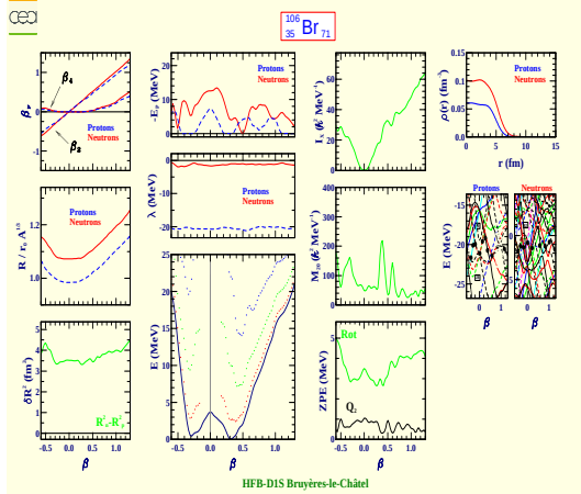
Bromine 106 (Z=35, N=71)
