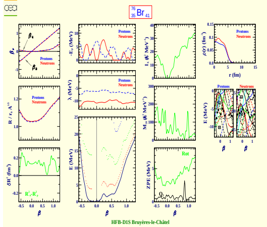
Bromine 76 (Z=35, N=41)
