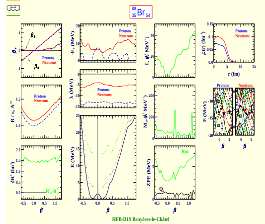
Bromine 89 (Z=35, N=54)
