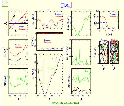
Bromine 116 (Z=35, N=81)
