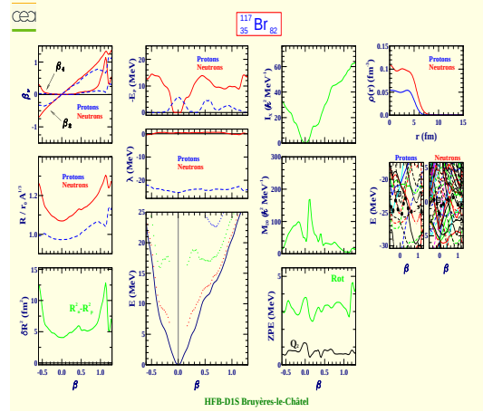
Brome 117 (Z=35, N=82)
