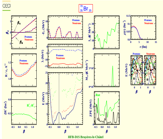
Brome 70 (Z=35, N=35)
