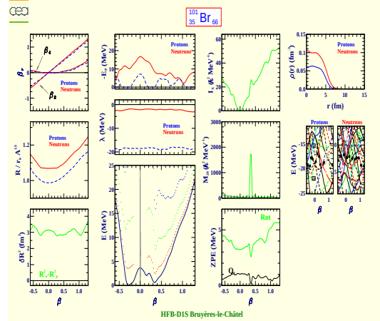
Brome 101 (Z=35, N=66)
