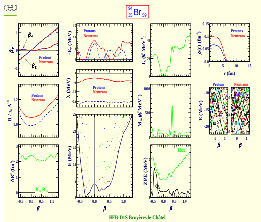
Brome 94 (Z=35, N=59)
