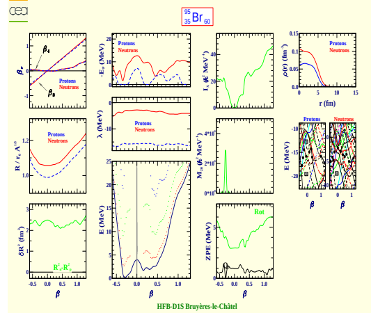
Brome 95 (Z=35, N=60)
