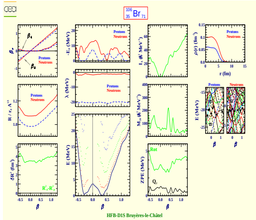
Brome 106 (Z=35, N=71)
