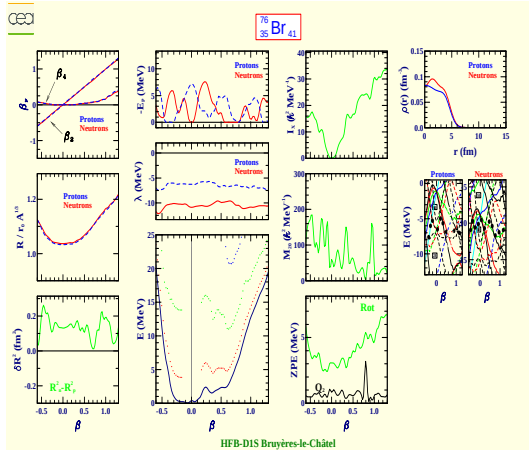
Brome 76 (Z=35, N=41)
