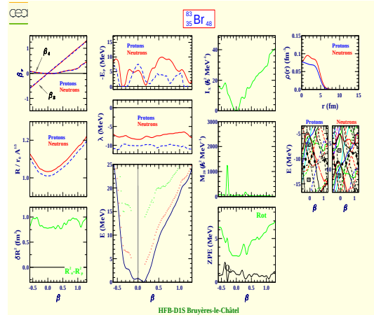
Brome 83 (Z=35, N=48)
