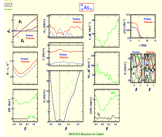
Arsenic 85 (Z=33, N=52)
