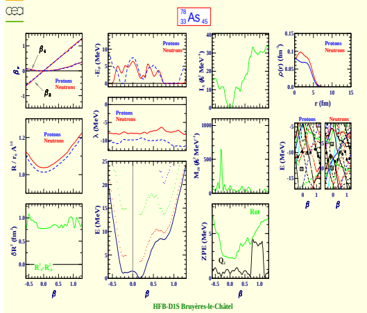
Arsenic 78 (Z=33, N=45)
