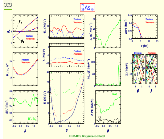
Arsenic 73 (Z=33, N=40)
