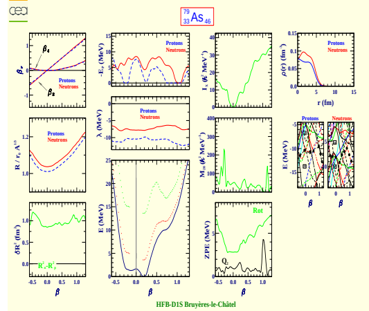
Arsenic 79 (Z=33, N=46)
