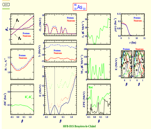
Arsenic 66 (Z=33, N=33)
