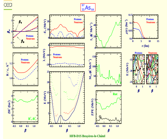
Arsenic 97 (Z=33, N=64)
