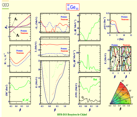
Germanium 82 (Z=32, N=50)
