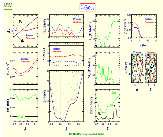
Germanium 77 (Z=32, N=45)
