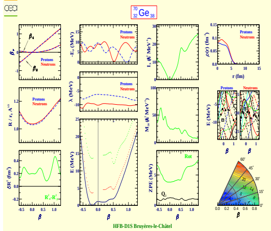
Germanium 70 (Z=32, N=38)
