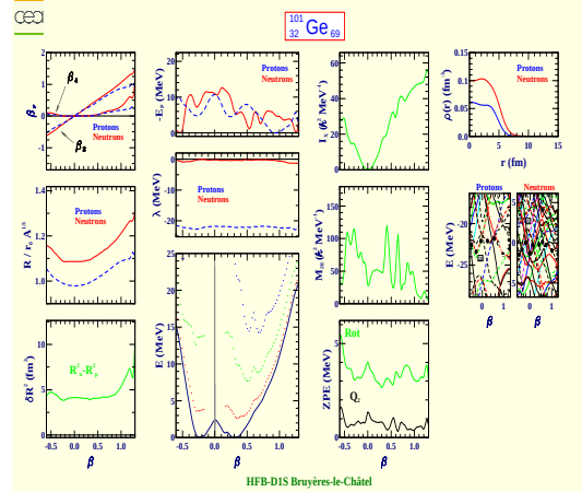
Germanium 101 (Z=32, N=69)
