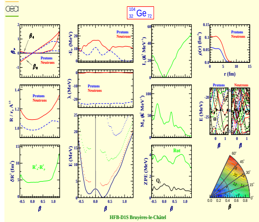
Germanium 104 (Z=32, N=72)
