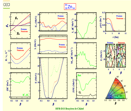
Zinc 84 (Z=30, N=54)
