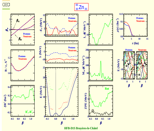
Zinc 65 (Z=30, N=35)
