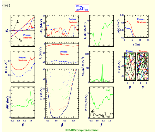
Zinc 89 (Z=30, N=59)
