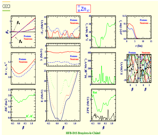
Zinc 77 (Z=30, N=47)
