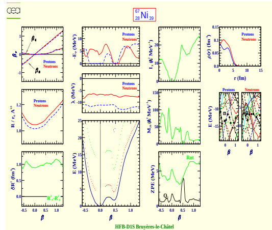
Nickel 67 (Z=28, N=39)
