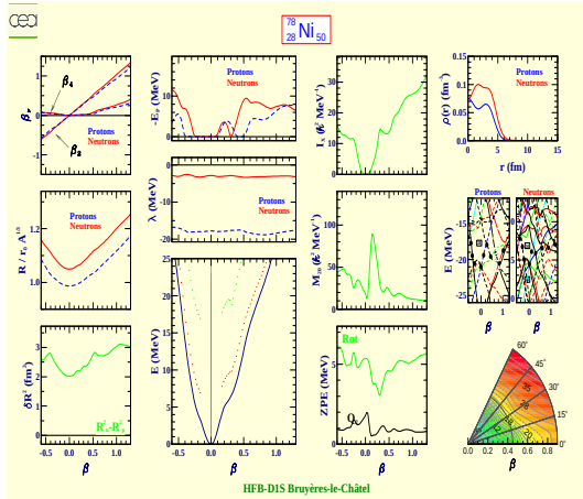
Nickel 78 (Z=28, N=50)
