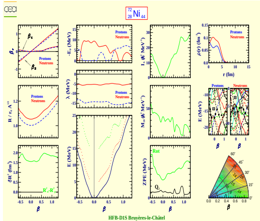
Nickel 72 (Z=28, N=44)
