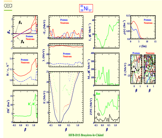
Nickel 85 (Z=28, N=57)
