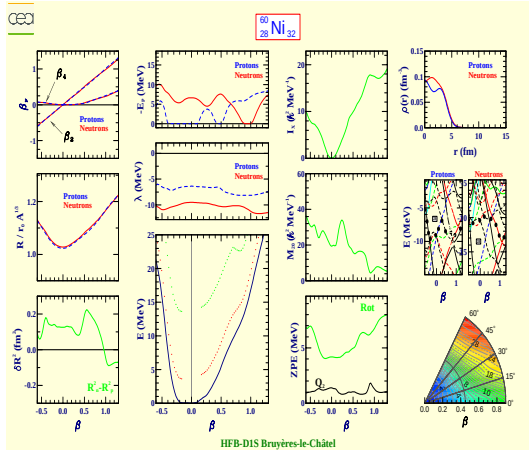
Nickel 60 (Z=28, N=32)
