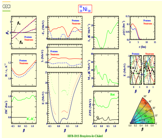
Nickel 66 (Z=28, N=38)
