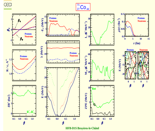
Cobalt 71 (Z=27, N=44)
