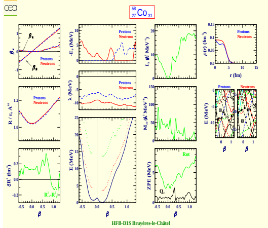
Cobalt 58 (Z=27, N=31)
