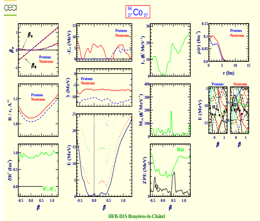
Cobalt 64 (Z=27, N=37)
