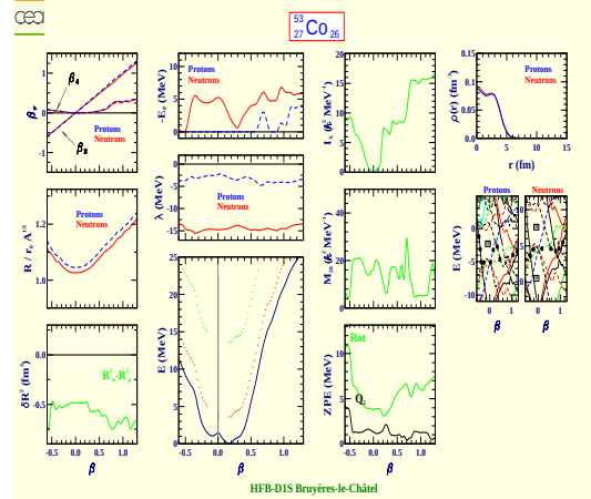
Cobalt 53 (Z=27, N=26)
