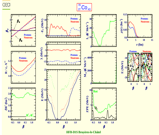
Cobalt 70 (Z=27, N=43)
