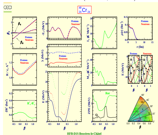
Chromium 48 (Z=24, N=24)
