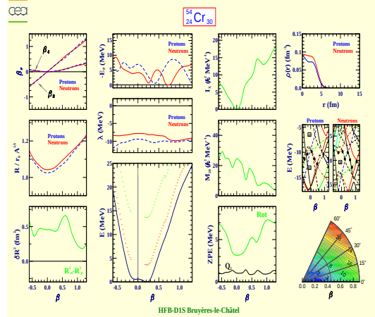
Chromium 54 (Z=24, N=30)
