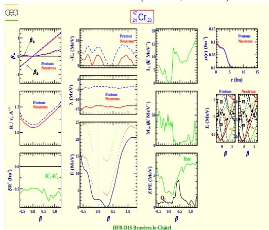
Chromium 47 (Z=24, N=23)
