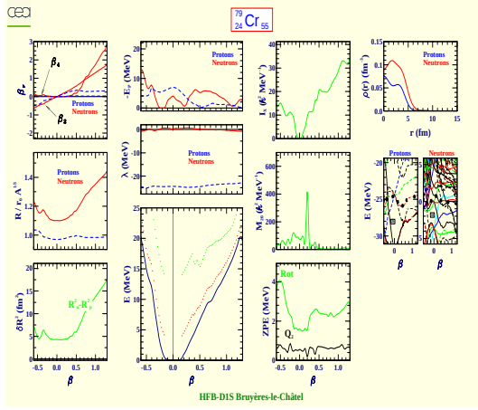
Chromium 79 (Z=24, N=55)
