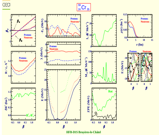
Chromium 59 (Z=24, N=35)
