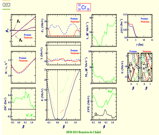
Chromium 53 (Z=24, N=29)
