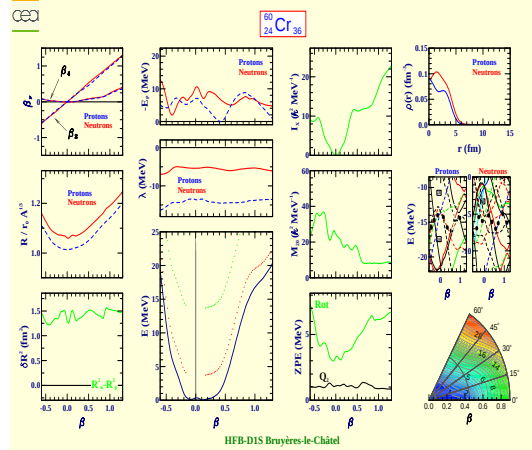
Chromium 60 (Z=24, N=36)
