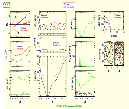
Calcium 57 (Z=20, N=37)
