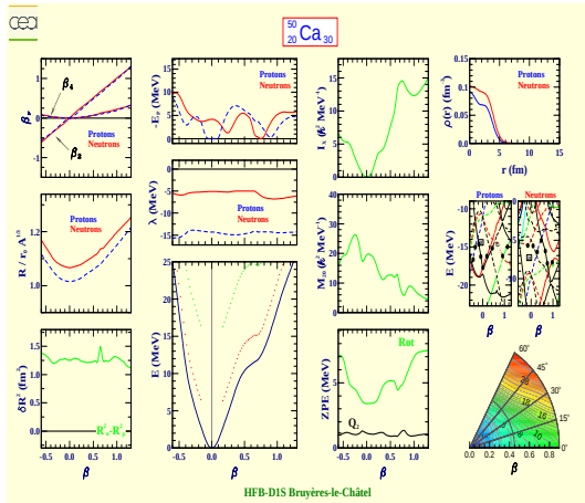
Calcium 50 (Z=20, N=30)
