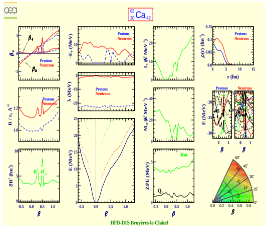
Calcium 62 (Z=20, N=42)
