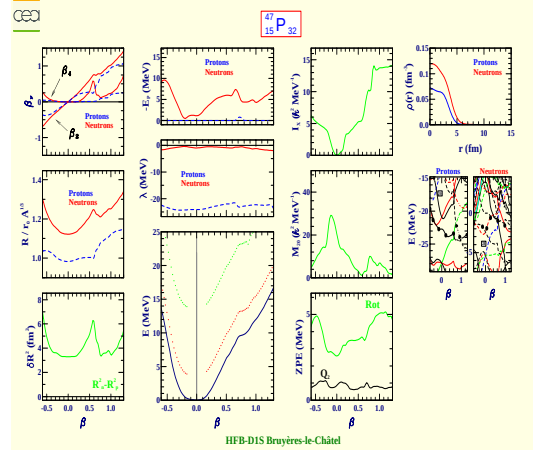
Phosphorus 47 (Z=15, N=32)
