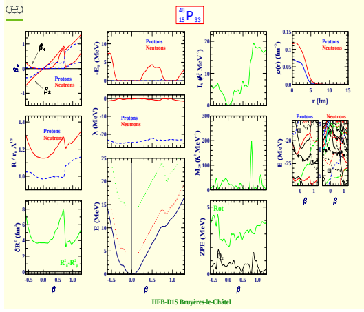
Phosphorus 48 (Z=15, N=33)
