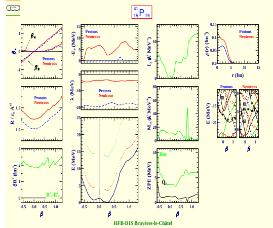
Phosphorus 41 (Z=15, N=26)
