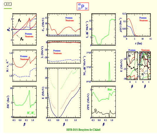
Phosphorus 49 (Z=15, N=34)
