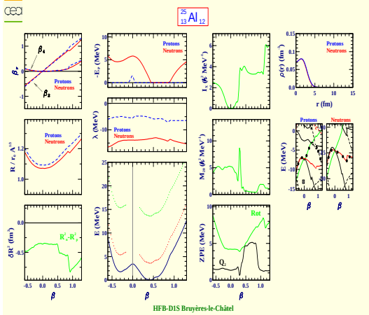
Aluminum 25 (Z=13, N=12)
