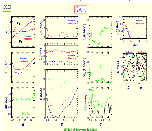
Aluminum 32 (Z=13, N=19)
