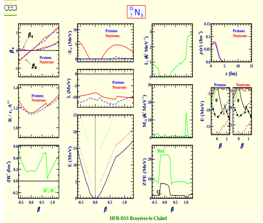
Nitrogen 15 (Z=7, N=8)
