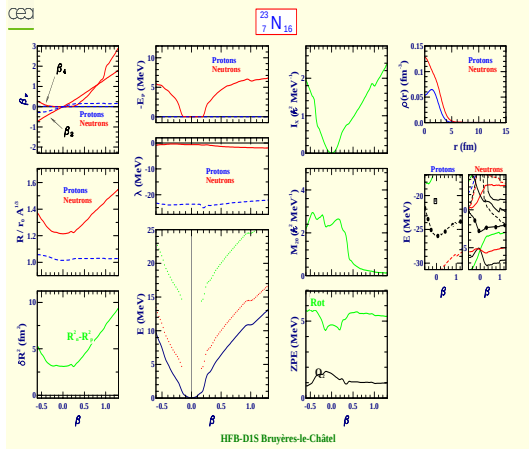
Nitrogen 23 (Z=7, N=16)
