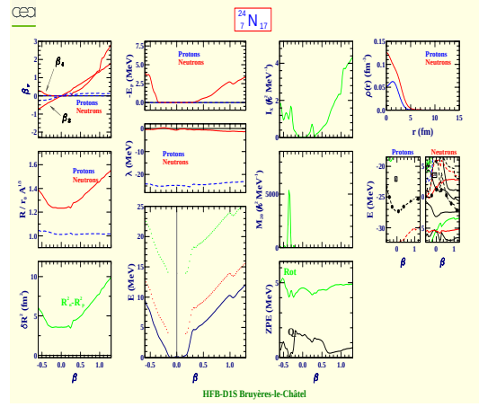
Nitrogen 24 (Z=7, N=17)
