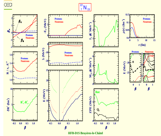
Nitrogen 22 (Z=7, N=15)
