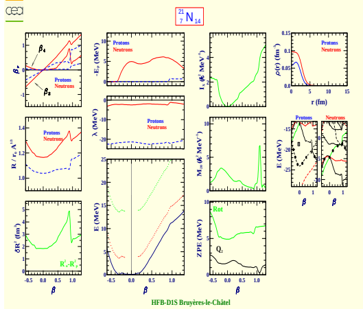
Nitrogen 21 (Z=7, N=14)
