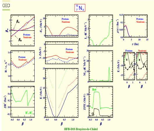
Azote 15 (Z=7, N=8)
