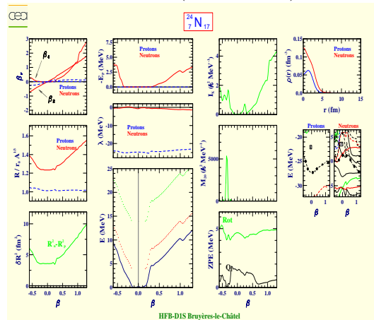
Azote 24 (Z=7, N=17)
