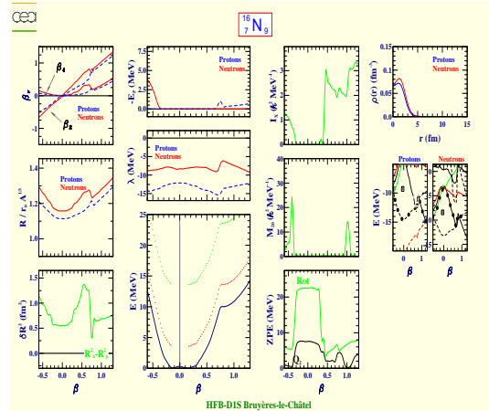
Azote 16 (Z=7, N=9)
