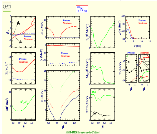
Azote 23 (Z=7, N=16)
