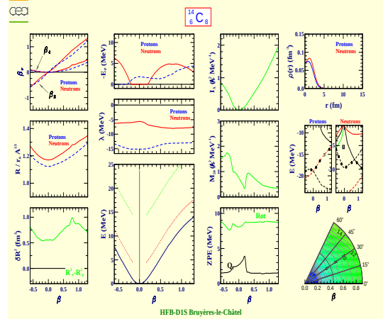
Carbon 14 (Z=6, N=8)
