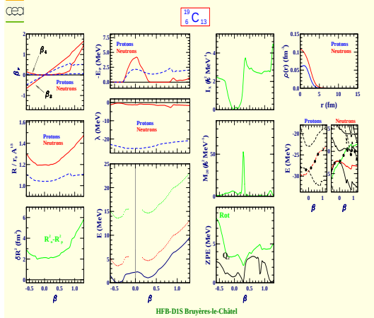
Carbon 19 (Z=6, N=13)
