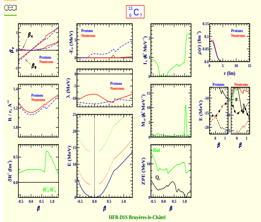
Carbon 13 (Z=6, N=7)
