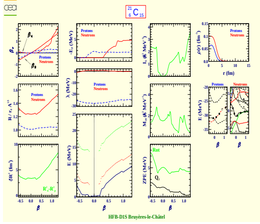
Carbon 21 (Z=6, N=15)
