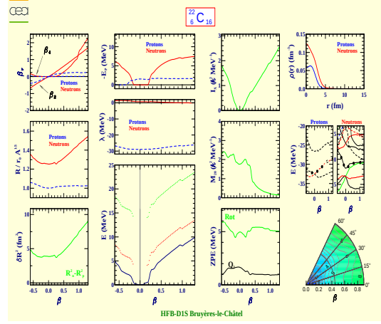
Carbon 22 (Z=6, N=16)
