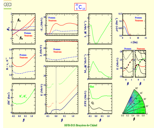
Carbon 20 (Z=6, N=14)
