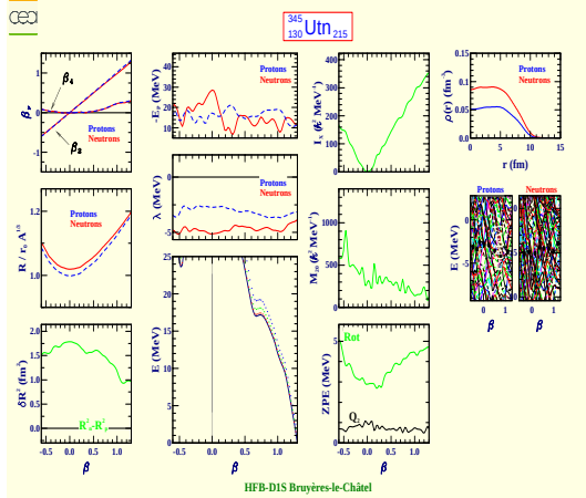
Untrinium 345 (Z=130, N=215)
