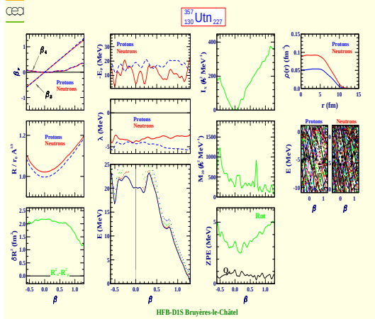
Untrinium 357 (Z=130, N=227)
