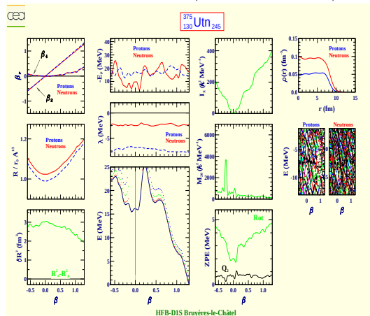
Untrinium 375 (Z=130, N=245)
