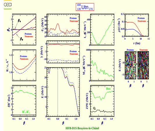
Untrinium 406 (Z=130, N=276)
