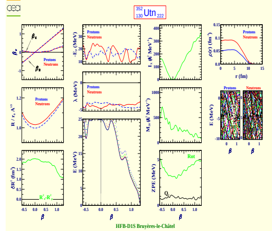
Untrinium 352 (Z=130, N=222)
