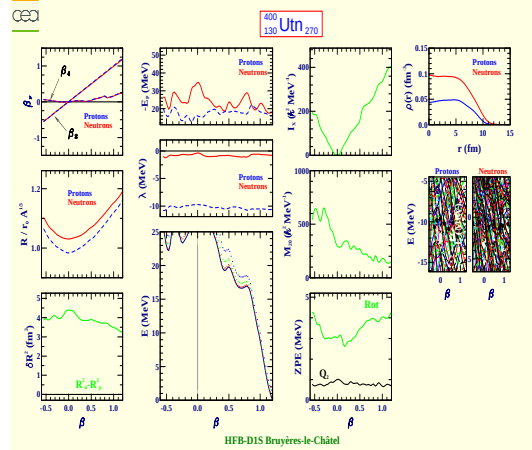
Untrinium 400 (Z=130, N=270)
