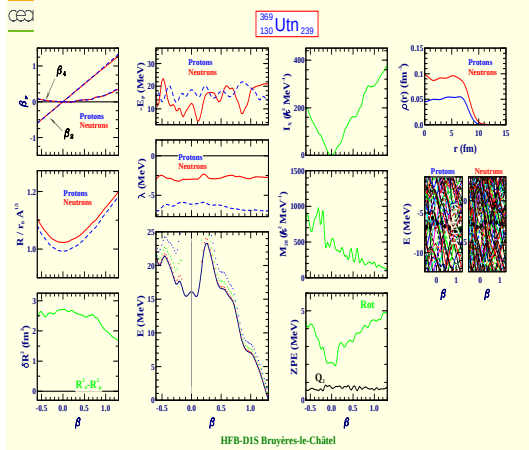
Untrinium 369 (Z=130, N=239)
