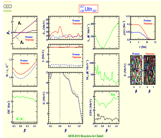
Untrinium 417 (Z=130, N=287)
