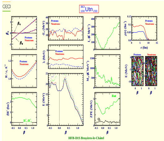
Untrinium 363 (Z=130, N=233)
