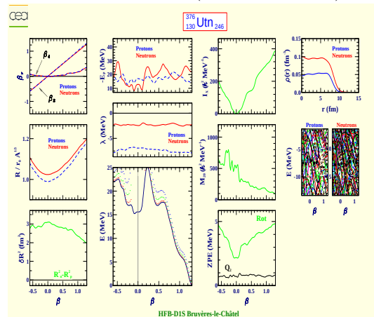
Untrinium 376 (Z=130, N=246)
