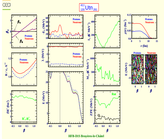
Untrinium 411 (Z=130, N=281)
