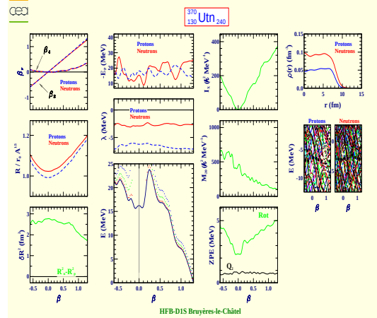
Untrinium 370 (Z=130, N=240)
