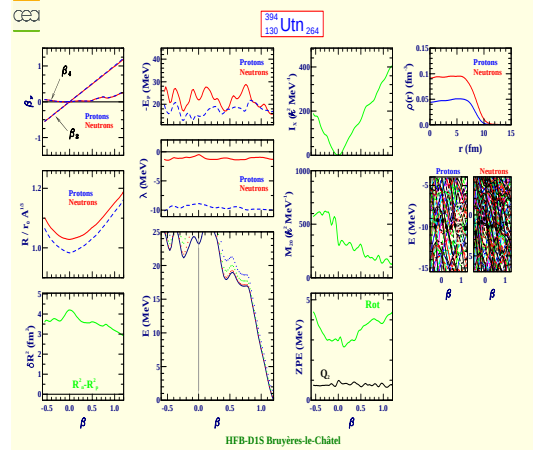
Untrinium 394 (Z=130, N=264)
