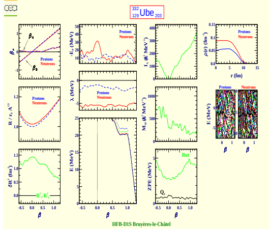
Unbiennium 332 (Z=129, N=203)
