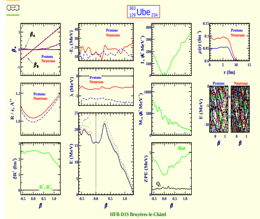
Unbiennium 363 (Z=129, N=234)
