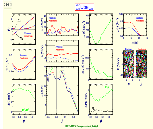
Unbiennium 357 (Z=129, N=228)
