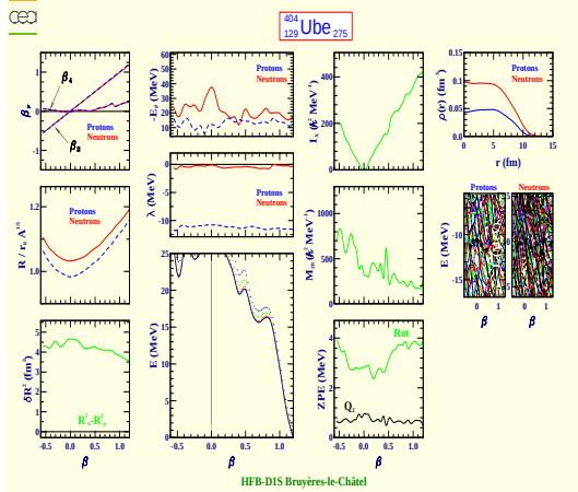
Unbiennium 404 (Z=129, N=275)
