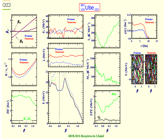
Unbiennium 362 (Z=129, N=233)
