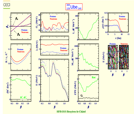
Unbiennium 369 (Z=129, N=240)
