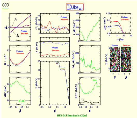
Unbiennium 326 (Z=129, N=197)
