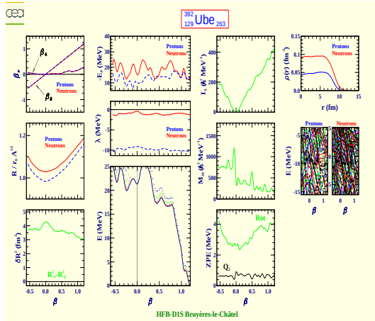
Unbiennium 392 (Z=129, N=263)
