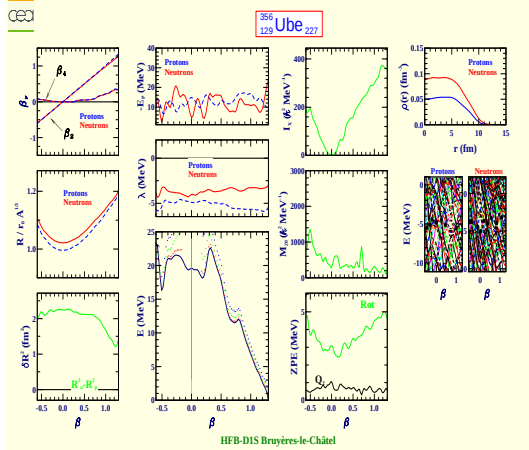
Unbiennium 356 (Z=129, N=227)
