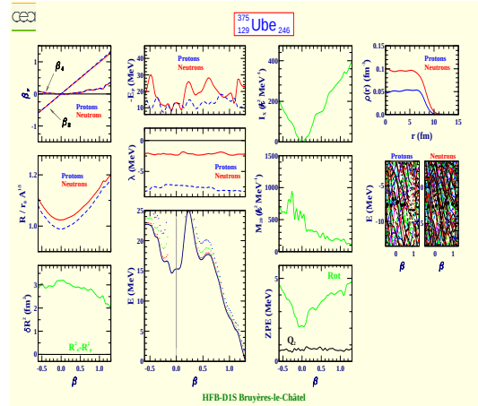
Unbiennium 375 (Z=129, N=246)
