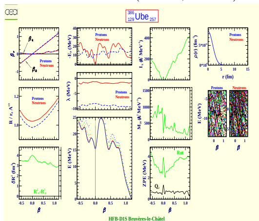
Unbiennium 386 (Z=129, N=257)
