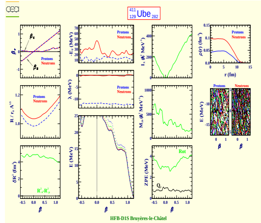
Unbiennium 411 (Z=129, N=282)
