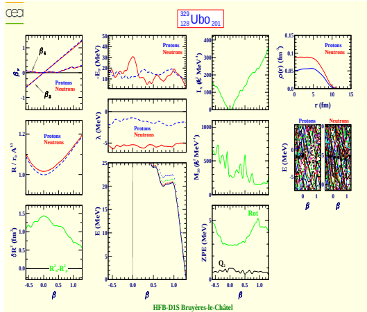
Unbioctium 329 (Z=128, N=201)
