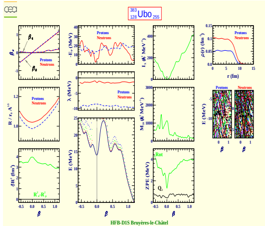
Unbioctium 383 (Z=128, N=255)
