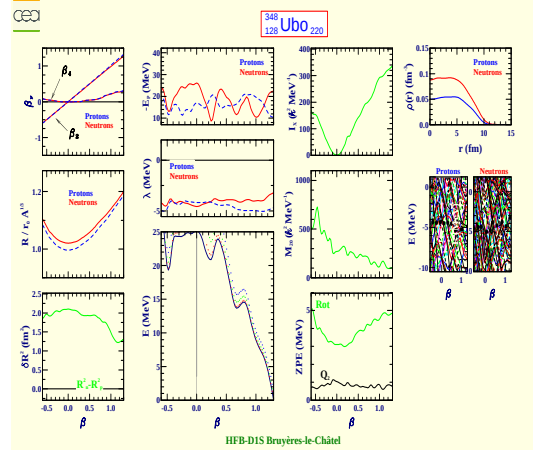
Unbioctium 348 (Z=128, N=220)
