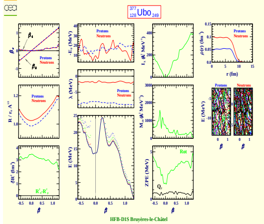
Unbioctium 377 (Z=128, N=249)
