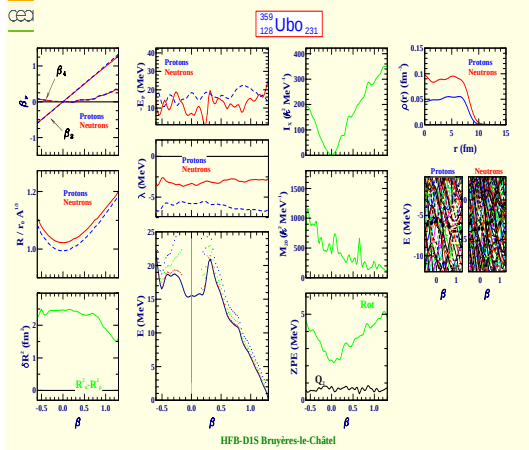
Unbioctium 359 (Z=128, N=231)
