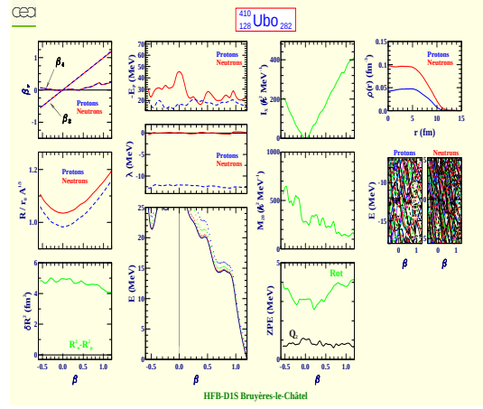
Unbioctium 410 (Z=128, N=282)
