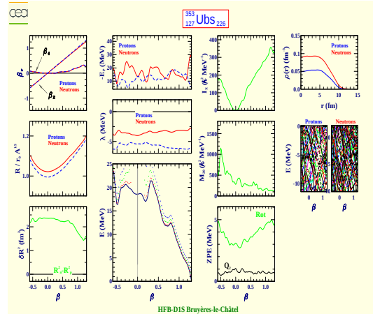
Unbseptium 353 (Z=127, N=226)
