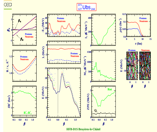
Unbseptium 371 (Z=127, N=244)
