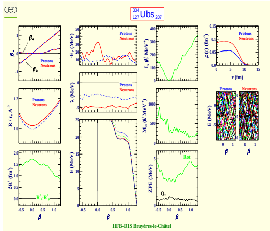
Unbseptium 334 (Z=127, N=207)
