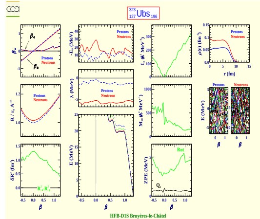
Unbseptium 323 (Z=127, N=196)
