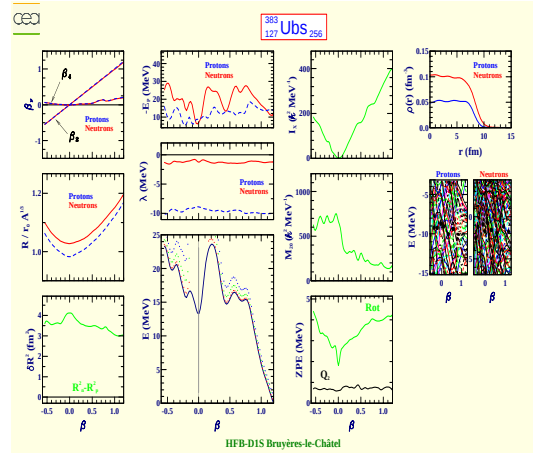
Unbiseptium 383 (Z=127, N=256)
