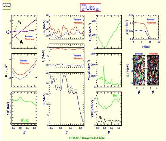
Unbseptium 388 (Z=127, N=261)
