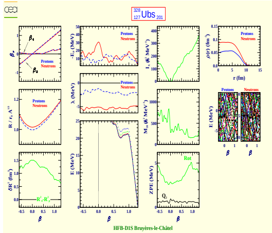
Unbseptium 328 (Z=127, N=201)
