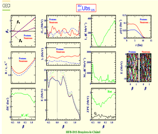
Unbseptium 352 (Z=127, N=225)
