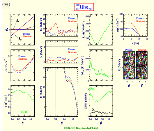
Unbseptium 340 (Z=127, N=213)
