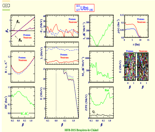
Unbseptium 322 (Z=127, N=195)
