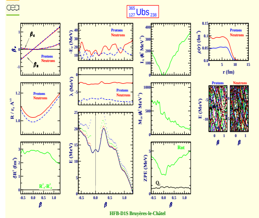
Unbiseptium 365 (Z=127, N=238)
