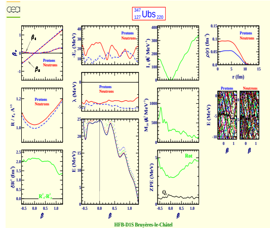
Unbseptium 347 (Z=127, N=220)
