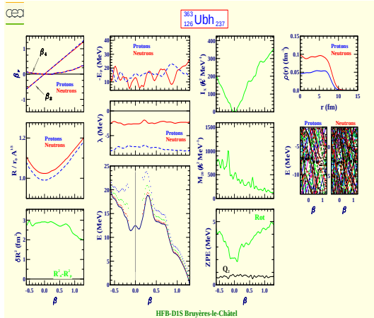
Unbihexium 363 (Z=126, N=237)
