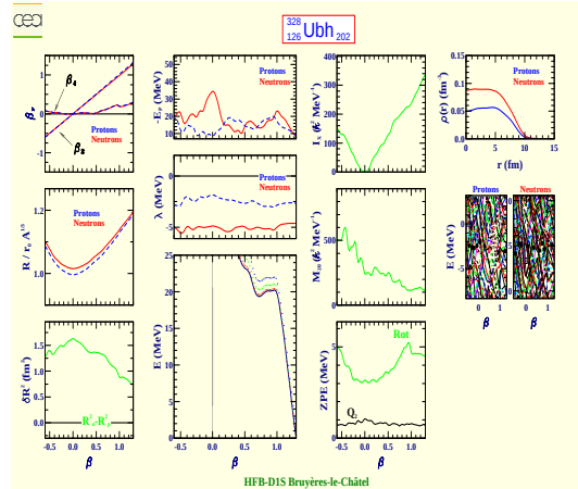
Unbihexium 328 (Z=126, N=202)
