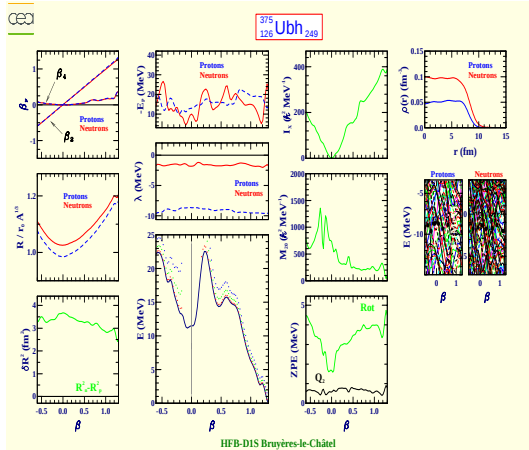
Unbihexium 375 (Z=126, N=249)
