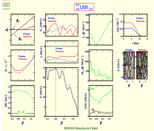
Unbihexium 345 (Z=126, N=219)
