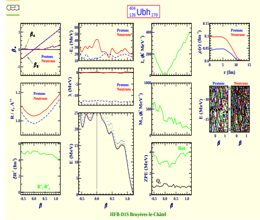
Unbihexium 404 (Z=126, N=278)
