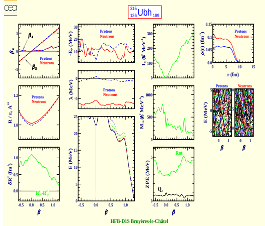
Unbihexium 315 (Z=126, N=189)
