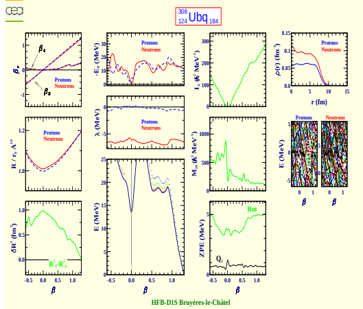
Unbiquadium 308 (Z=124, N=184)
