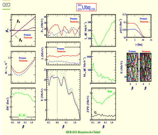
Unbiquadium 344 (Z=124, N=220)
