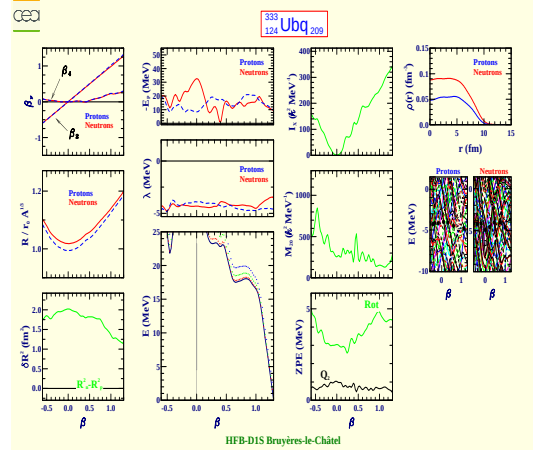
Unbiquadium 333 (Z=124, N=209)
