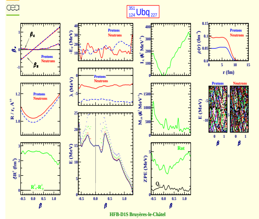
Unbiquadium 351 (Z=124, N=227)
