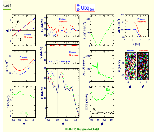
Unbiquadium 384 (Z=124, N=260)
