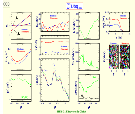
Unbiquadium 363 (Z=124, N=239)
