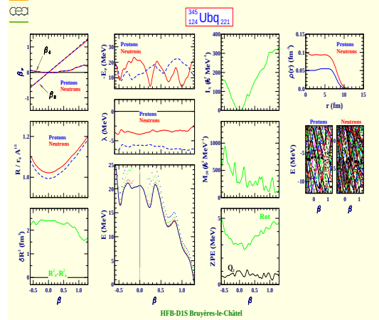
Unbiquadium 345 (Z=124, N=221)
