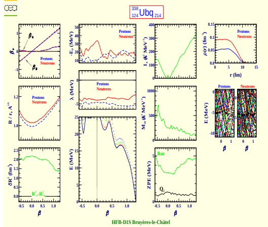
Unbiquadium 338 (Z=124, N=214)
