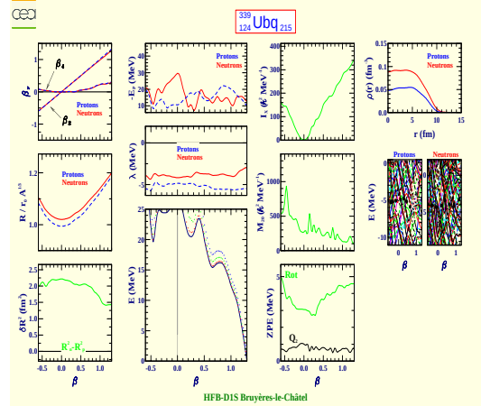
Unbiquadium 339 (Z=124, N=215)
