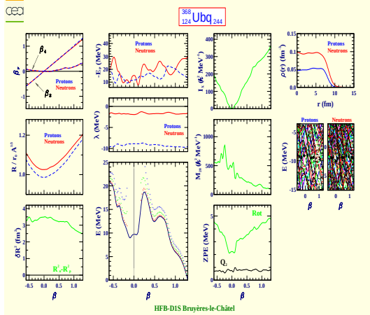
Unbiquadium 368 (Z=124, N=244)
