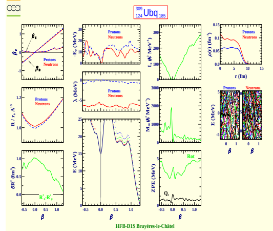
Unbiquadium 309 (Z=124, N=185)
