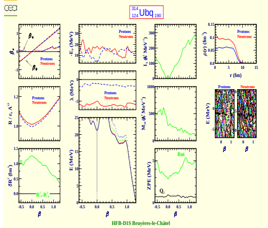
Unbiquadium 314 (Z=124, N=190)
