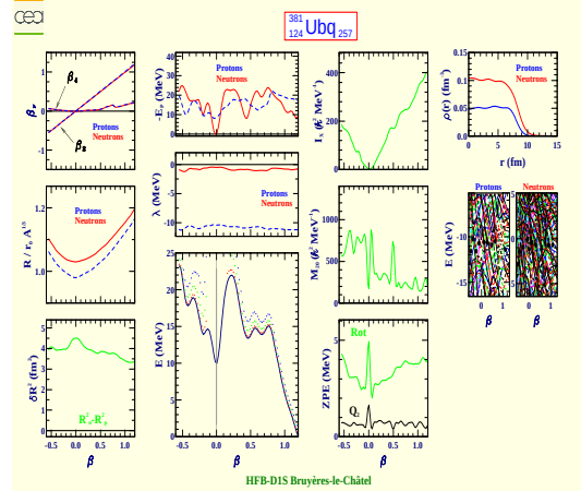
Unbiquadium 381 (Z=124, N=257)
