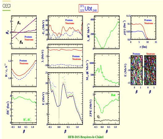
Unbitrium 371 (Z=123, N=248)
