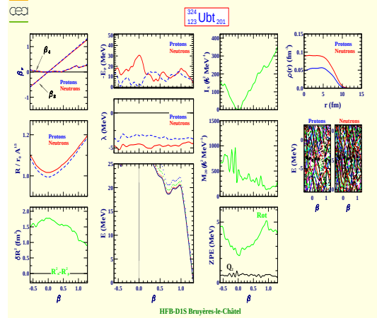
Unbitrium 324 (Z=123, N=201)
