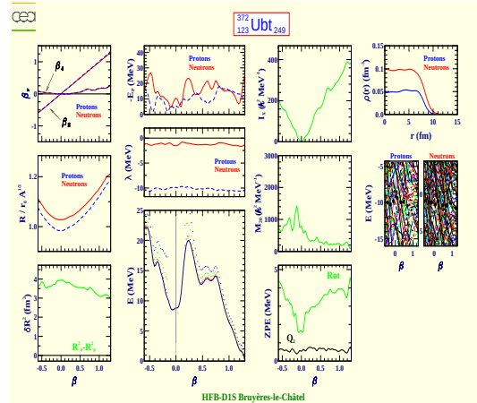
Unbitrium 372 (Z=123, N=249)
