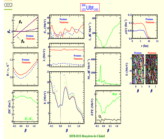
Unbitrium 366 (Z=123, N=243)
