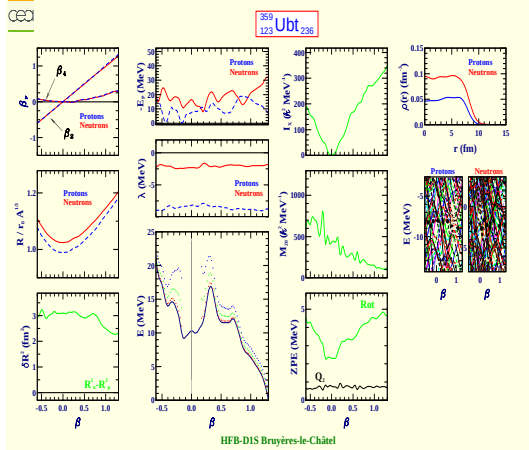
Unbitrium 359 (Z=123, N=236)
