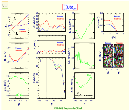
Unbitrium 329 (Z=123, N=206)
