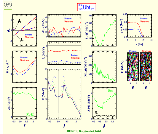
Unbitrium 354 (Z=123, N=231)
