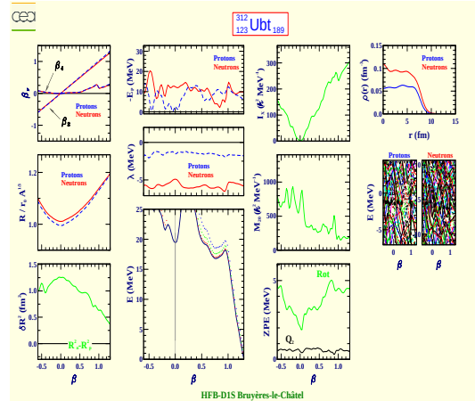
Unbitrium 312 (Z=123, N=189)
