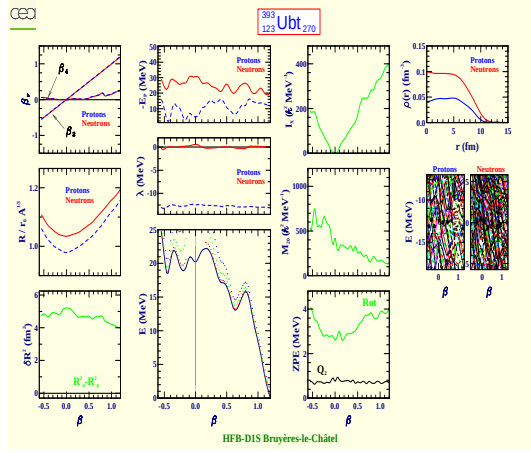
Unbitrium 393 (Z=123, N=270)
