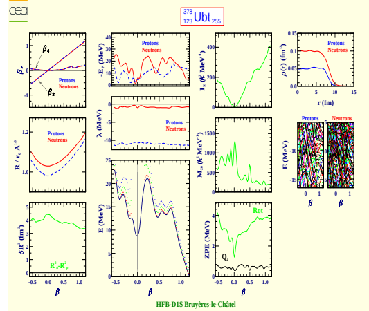
Unbitrium 378 (Z=123, N=255)
