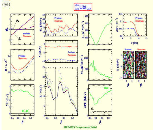
Unbitrium 365 (Z=123, N=242)
