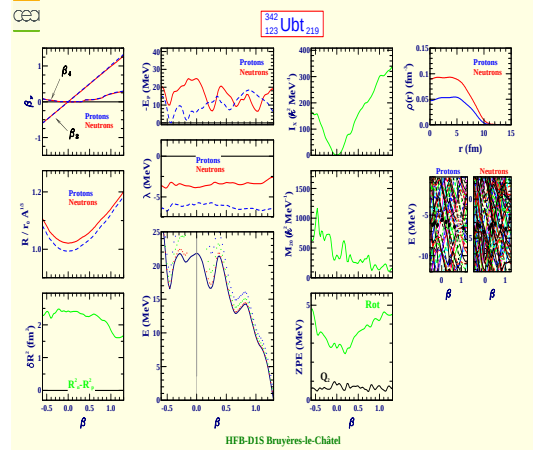
Unbitrium 342 (Z=123, N=219)
