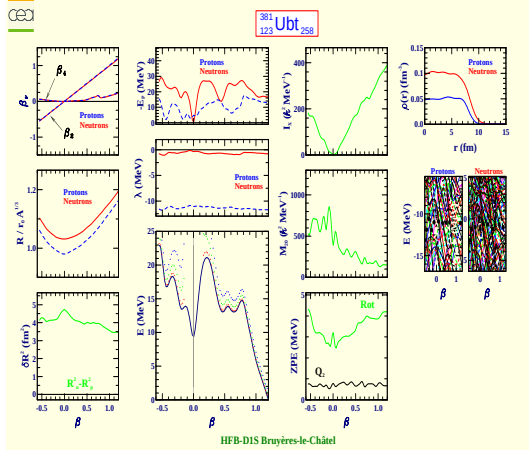
Unbitrium 381 (Z=123, N=258)
