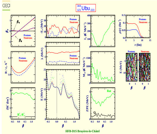
Unbiunium 344 (Z=121, N=223)
