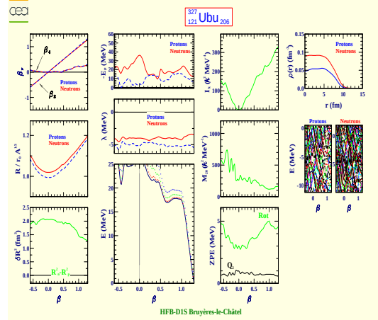
Unbiunium 327 (Z=121, N=206)
