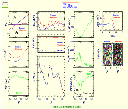
Unbiunium 374 (Z=121, N=253)
