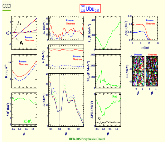
Unbiunium 368 (Z=121, N=247)
