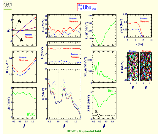
Unbiunium 357 (Z=121, N=236)
