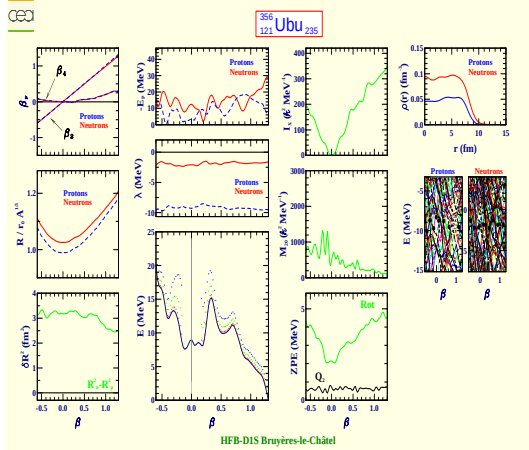
Unbiunium 356 (Z=121, N=235)
