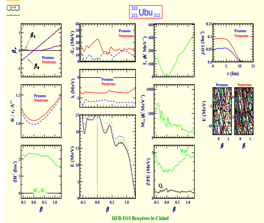
Unbiunium 333 (Z=121, N=212)
