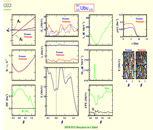
Unbiunium 297 (Z=121, N=176)
