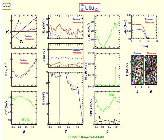
Unbiunium 314 (Z=121, N=193)
