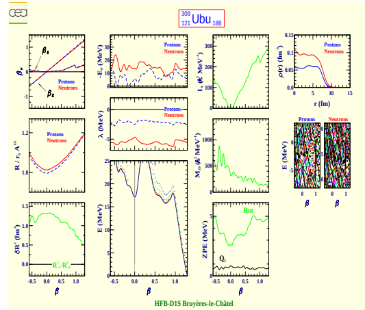
Unbiunium 309 (Z=121, N=188)
