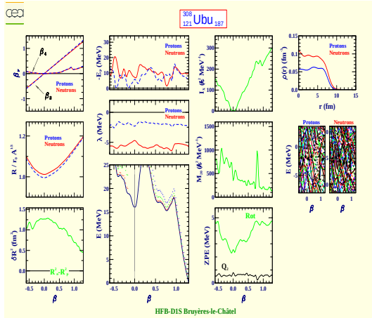
Unbiunium 308 (Z=121, N=187)
