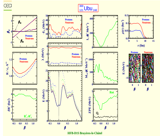
Unbiunium 369 (Z=121, N=248)
