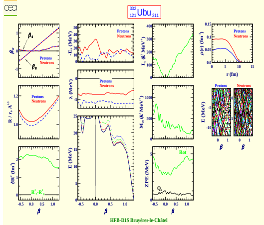
Unbiunium 332 (Z=121, N=211)
