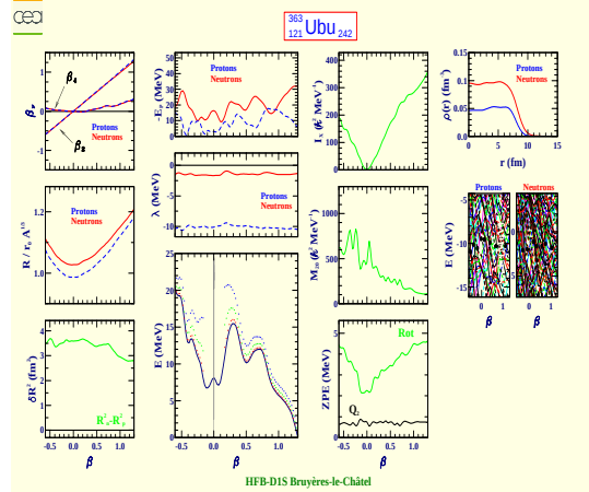
Unbiunium 363 (Z=121, N=242)
