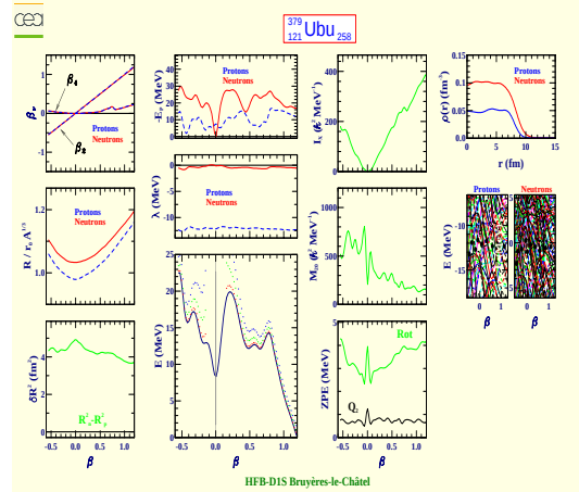
Unbiunium 379 (Z=121, N=258)
