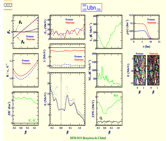
Unbinilium 355 (Z=120, N=235)
