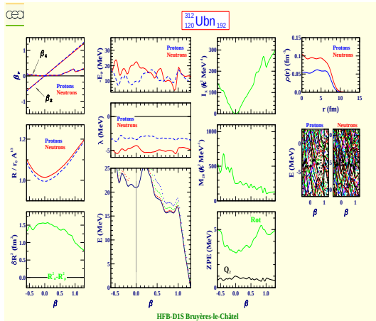
Unbinilium 312 (Z=120, N=192)
