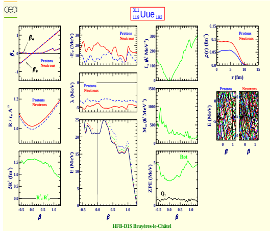
Ununennium 311 (Z=119, N=192)
