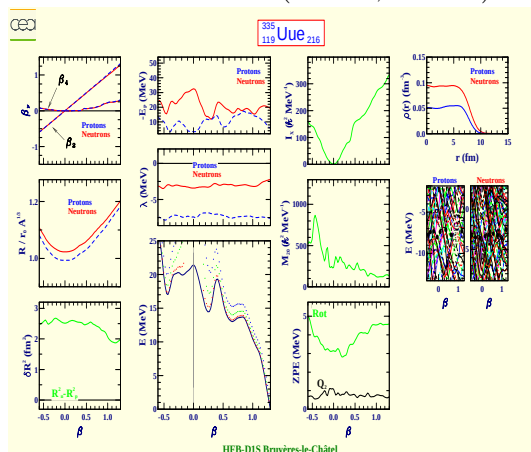
Ununennium 335 (Z=119, N=216)
