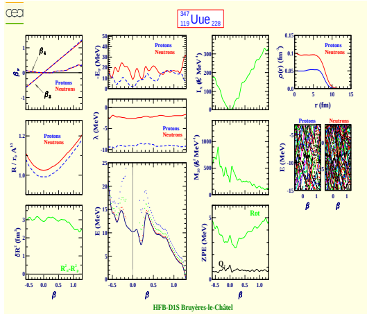
Ununennium 347 (Z=119, N=228)
