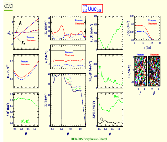
Ununennium 324 (Z=119, N=205)
