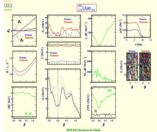
Ununennium 366 (Z=119, N=247)
