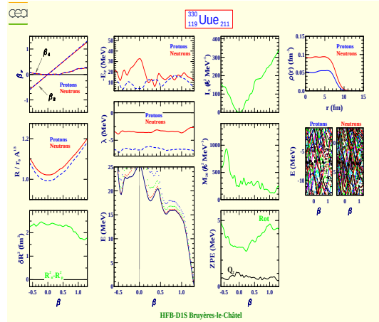
Ununennium 330 (Z=119, N=211)
