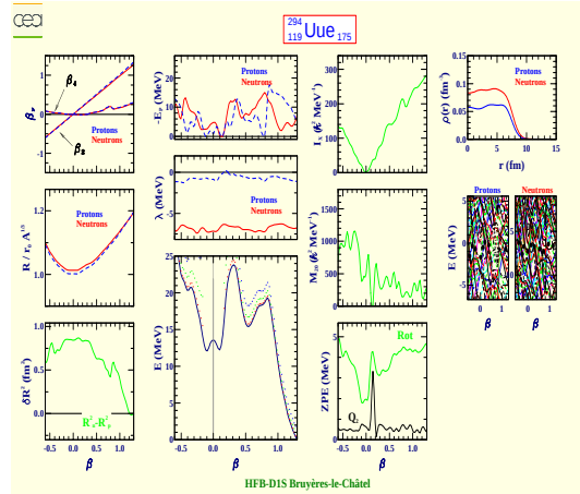
Ununennium 294 (Z=119, N=175)
