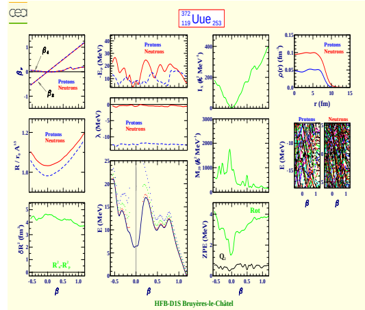
Ununennium 372 (Z=119, N=253)
