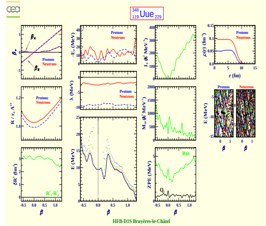
Ununennium 348 (Z=119, N=229)
