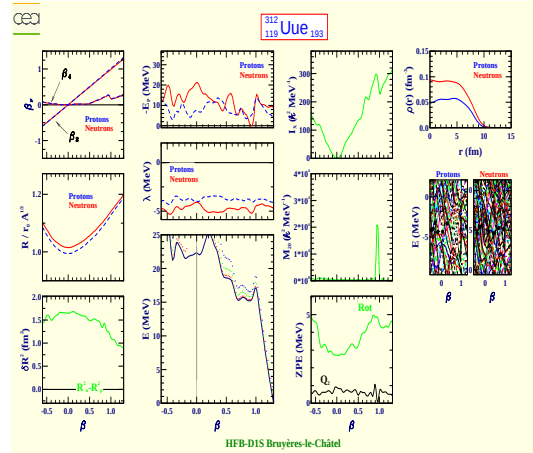
Ununennium 312 (Z=119, N=193)
