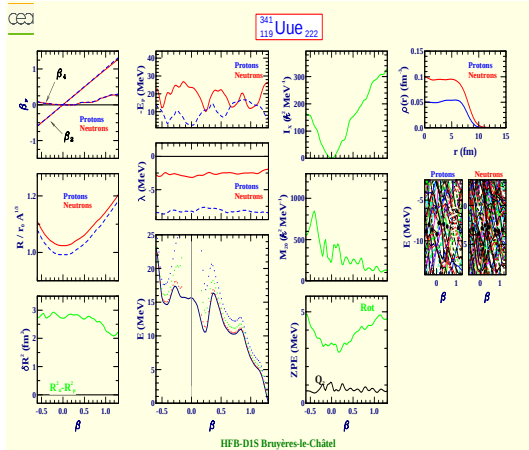
Ununennium 341 (Z=119, N=222)
