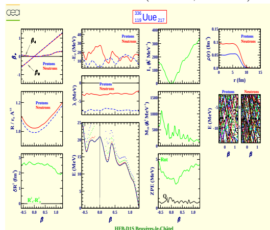
Ununennium 336 (Z=119, N=217)
