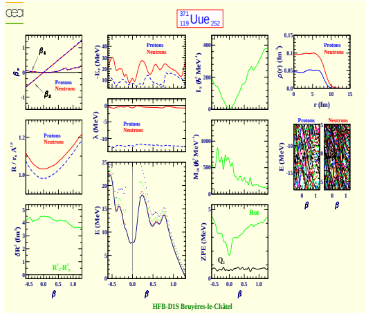
Ununennium 371 (Z=119, N=252)
