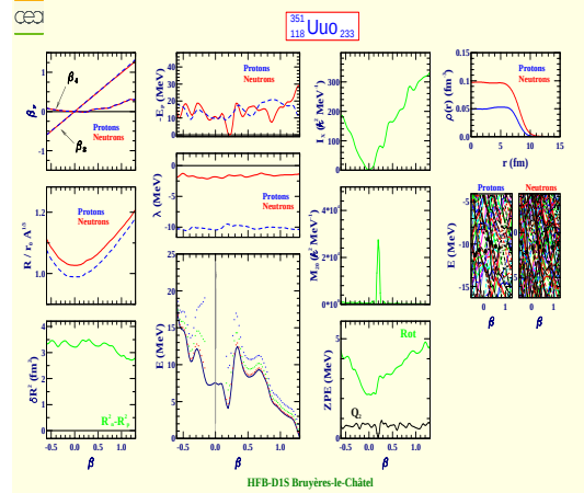
Ununoctium 351 (Z=118, N=233)
