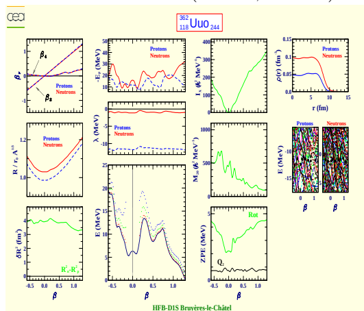
Ununoctium 362 (Z=118, N=244)
