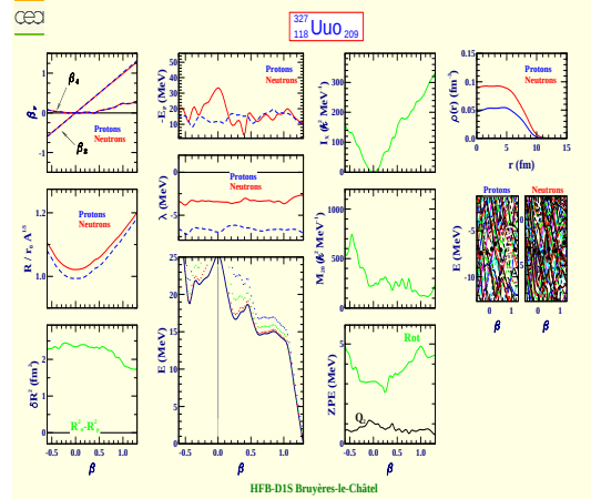
Ununoctium 327 (Z=118, N=209)
