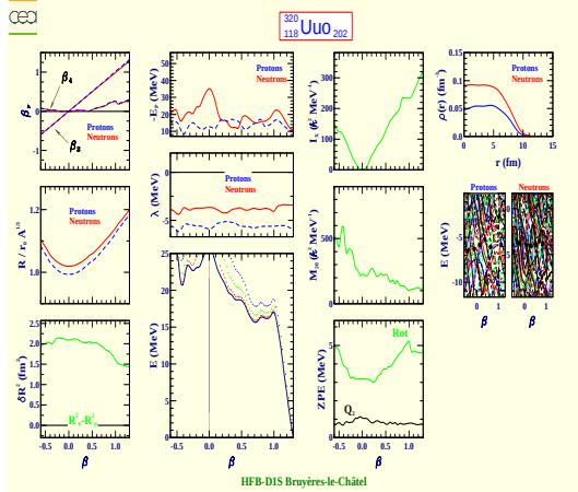
Ununoctium 320 (Z=118, N=202)
