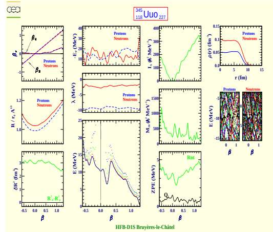
Ununoctium 345 (Z=118, N=227)
