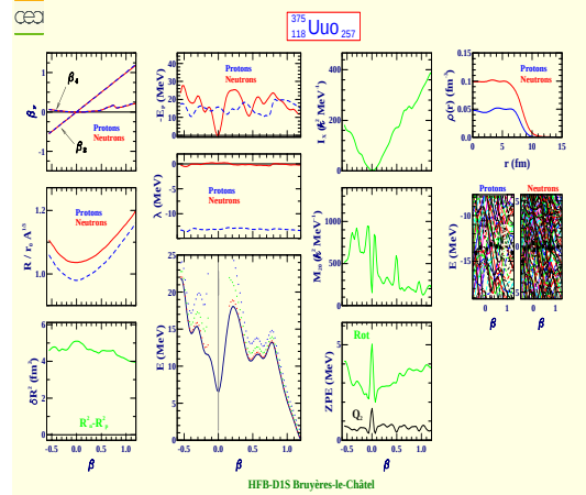
Ununoctium 375 (Z=118, N=257)
