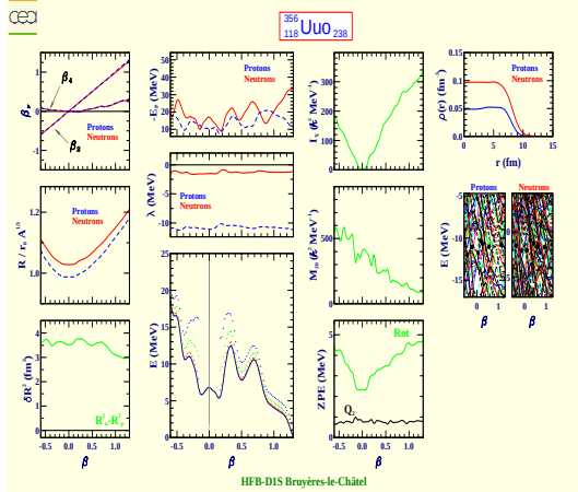
Ununoctium 356 (Z=118, N=238)
