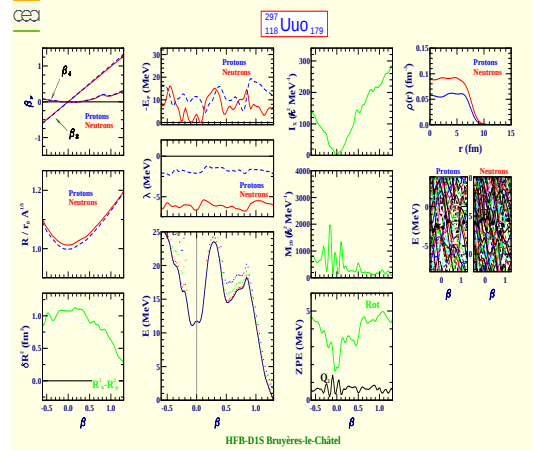
Ununoctium 297 (Z=118, N=179)
