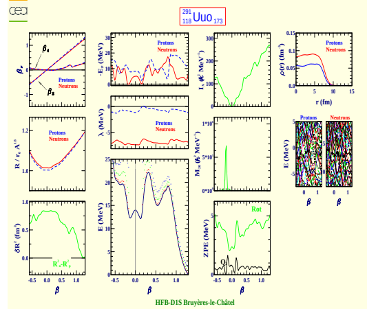
Ununoctium 291 (Z=118, N=173)
