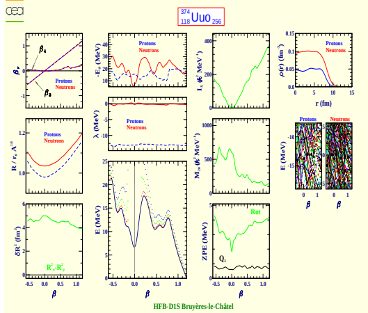
Ununoctium 374 (Z=118, N=256)
