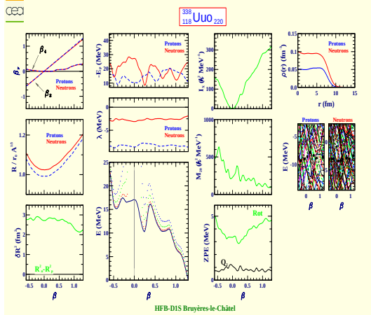
Ununoctium 338 (Z=118, N=220)
