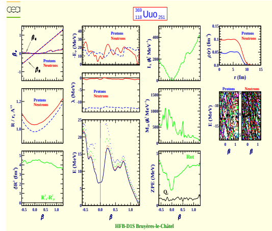
Ununoctium 369 (Z=118, N=251)
