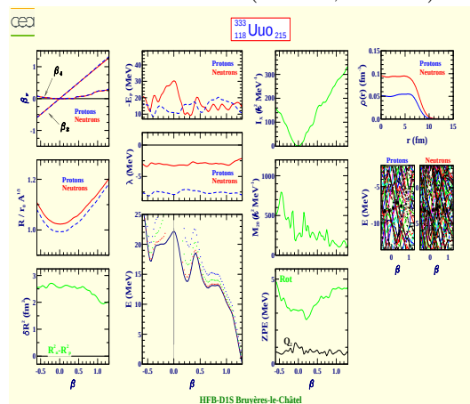
Ununoctium 333 (Z=118, N=215)
