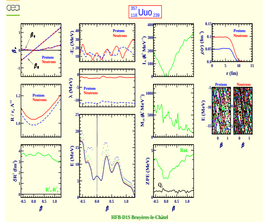
Ununoctium 357 (Z=118, N=239)
