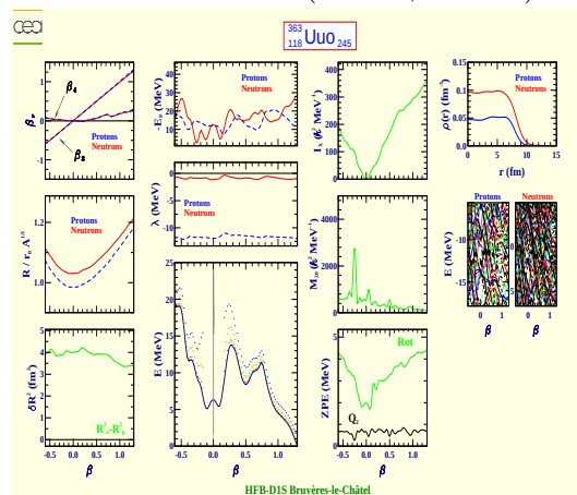
Ununoctium 363 (Z=118, N=245)
