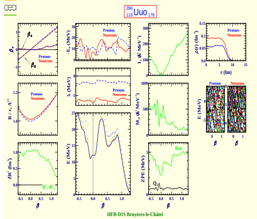
Ununoctium 296 (Z=118, N=178)
